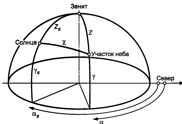
Рисунок 1 — Углы, определяющие положение солнца и участка неба
