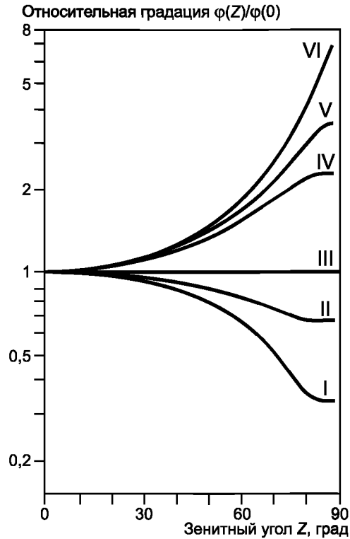
Рисунок 2 — Группы функций типowego изменения яркости при изменении защитного угла
