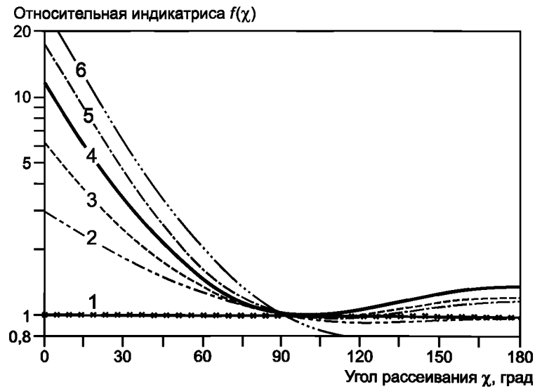
Рисунок 3 — Группы функций типовой индикатрисы яркости неба
