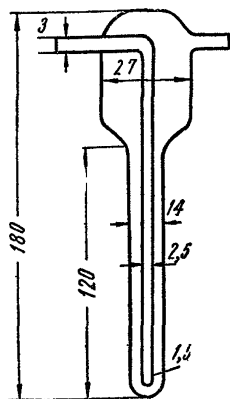
Рис. 5. Поглощительный прибор Зайцева.
