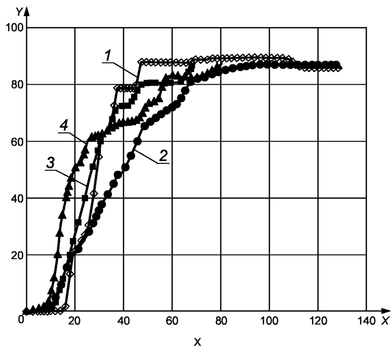
Рисунок А.7 — Результаты испытания на биоразложение трех образцов порошка ПКЛ [средний размер частиц — (180,7 \pm 76,8) мкм] с использованием закрытого респирометра при 25 °С в соответствии с ГОСТ Р 57219 (в качестве контрольного материала использовали порошок целлюлозы с размером частиц менее 20 мкм)
