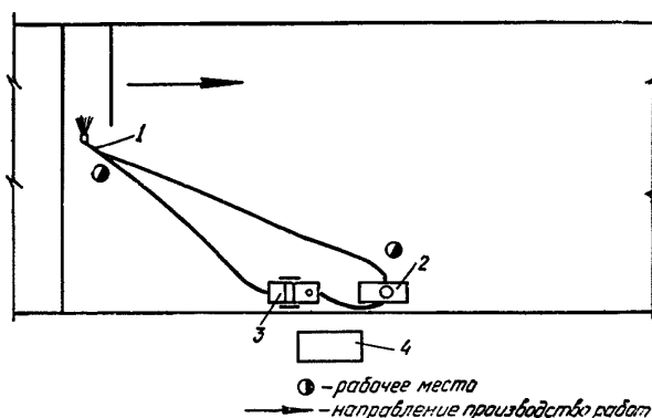
Рис. Устройство защитного слоя краской БТ-177 — пистолет-распылитель; 2 — красконагнетательный бачок; 3 — компрессор СО-2; 4 — подъемник УПСР
