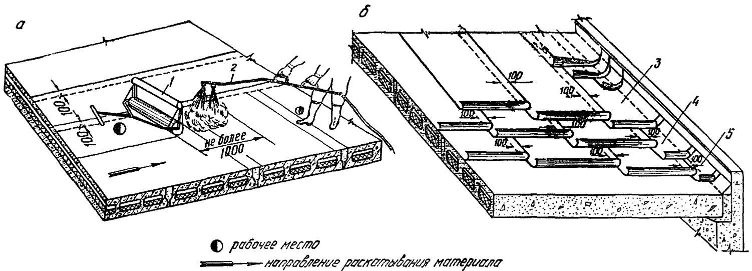
Рис. 3. Схема устройства рулонной кровли
