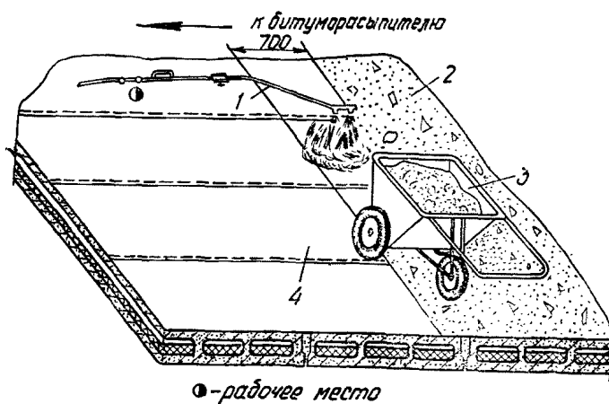
Рис. 4. Устройство защитного слоя с помощью бункера на пневмоходу
