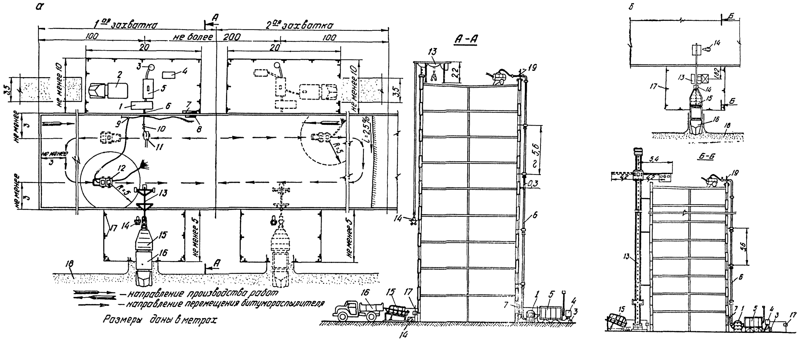
Рис. 2. Схема производства работ
