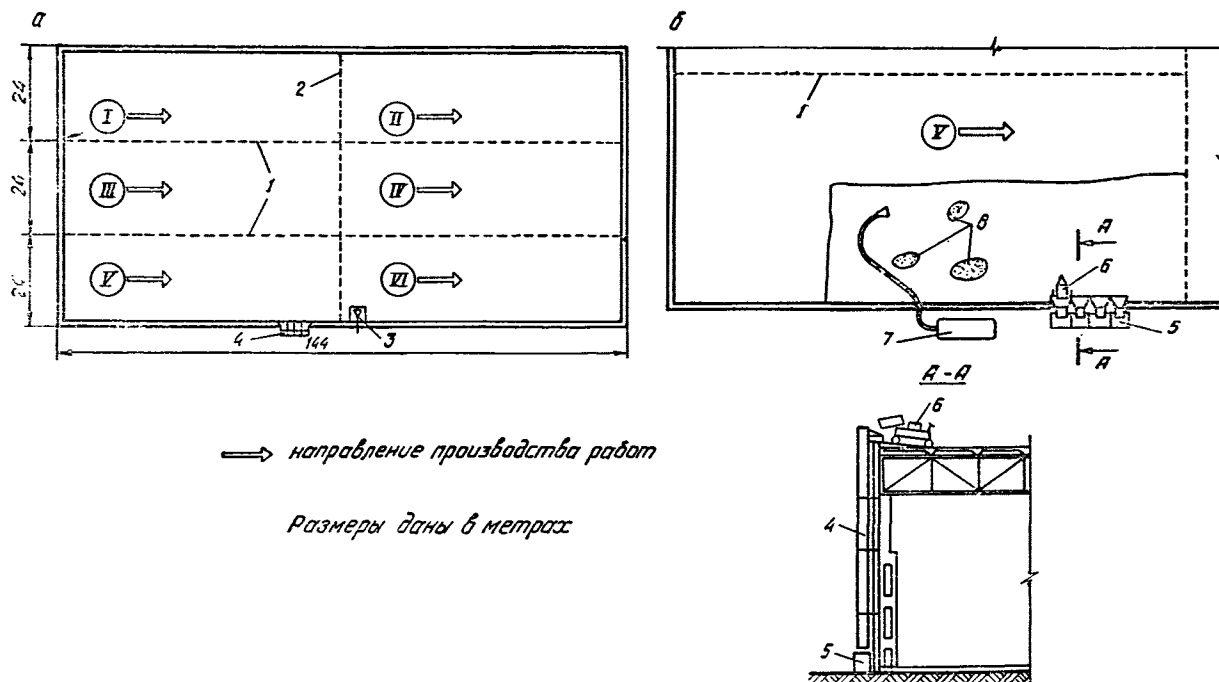
Рис. Организация работ при подготовке поверхности покрытия
