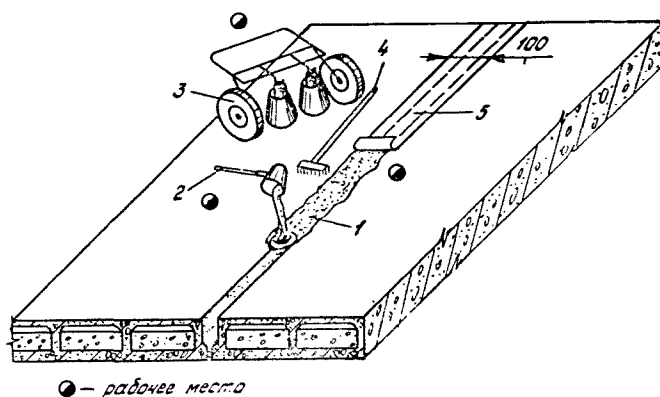
Рис. 4. Деталь оклейки стыка
