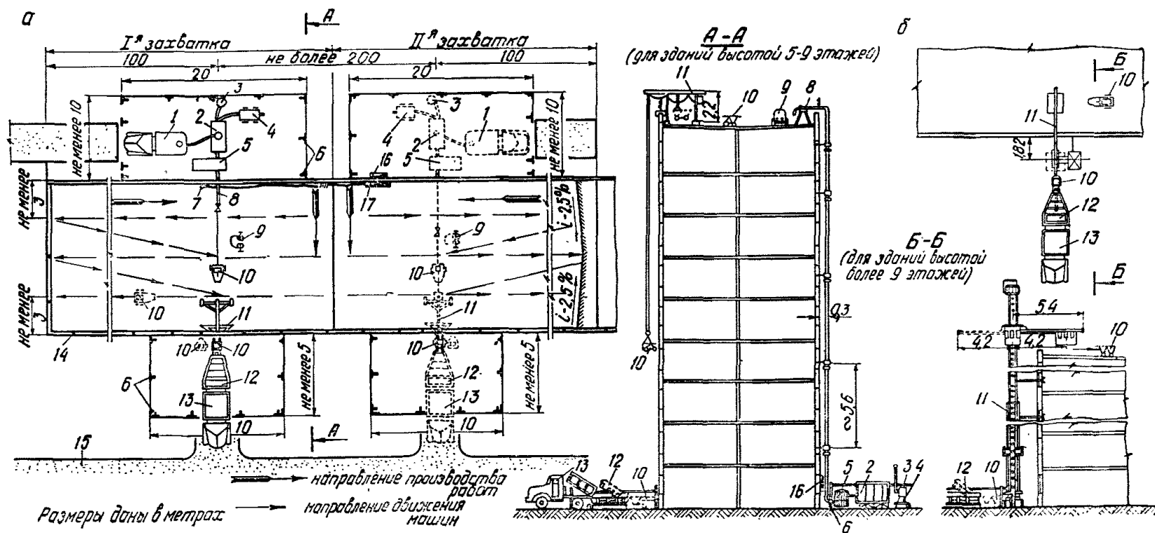
Рис. 1. Схема производства работ при заделке стыков плит покрытия в жилых зданиях
