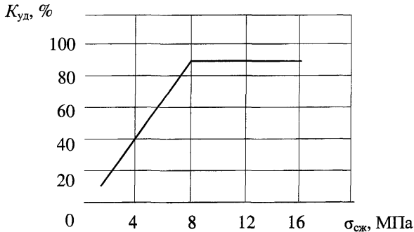
Рис. 1. График зависимости K_{уд} от \sigma_{сж}
