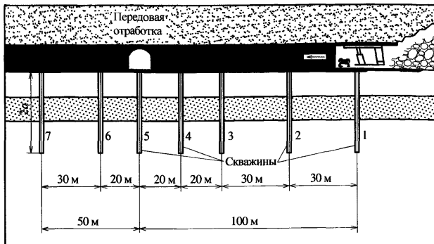
Рис. 1. Схема заложения геолого-разведочных скважин в районе передовой выработки
