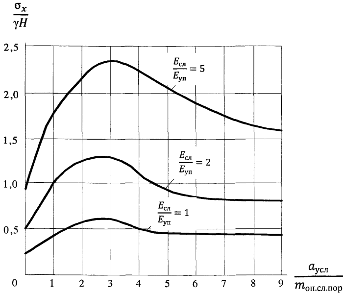
Рис. 3. Номограмма для определения \sigma_x в опасном слое:
