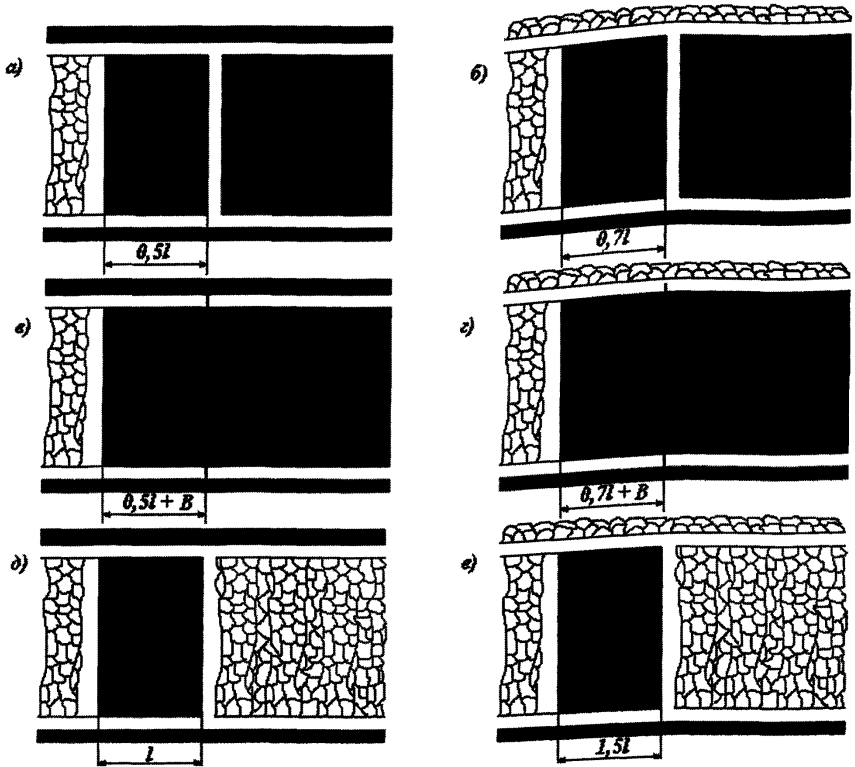
Рис. 1. Схемы определения d :
