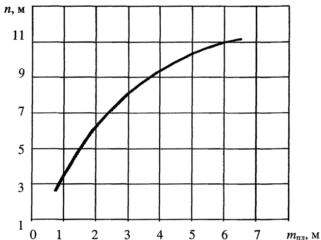
Рис. 3. Номограмма для определения ширины защитной зоны в краевой части угольного пласта
