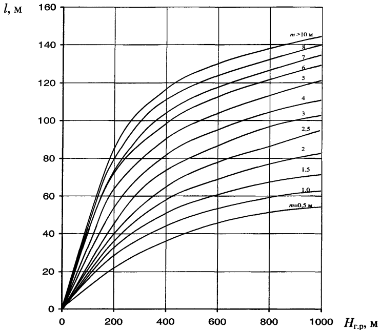
Рис. 2. Номограмма для определения ширины зоны опорного давления:
