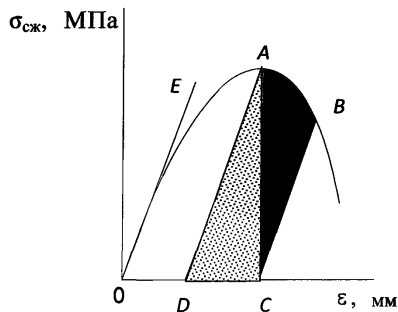
Рис. 2. График зависимости \sigma_{сж} от \epsilon
