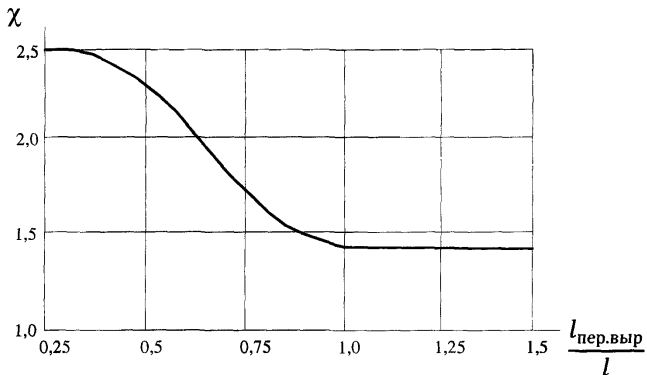
Рис. 2. Номограмма для определения \chi :
