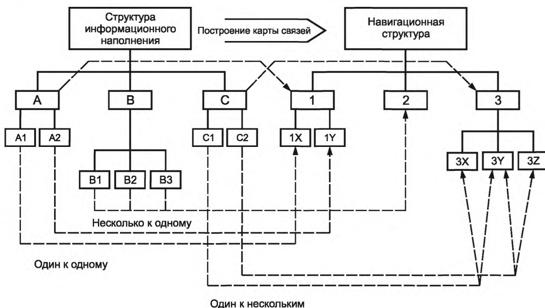
Рисунок 5 — Пример карты связей частей информационного наполнения и сегментов представления информации
