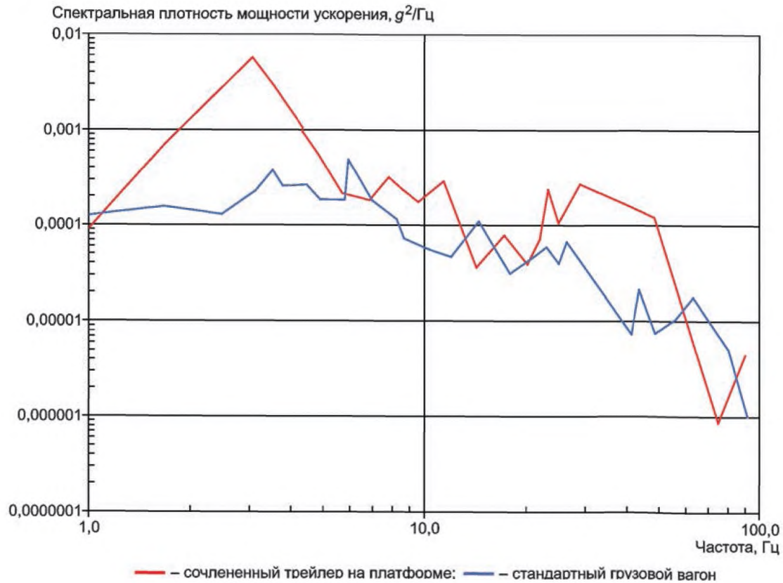
Рисунок 37 — Результаты измерений вибрации, по данным [12]
