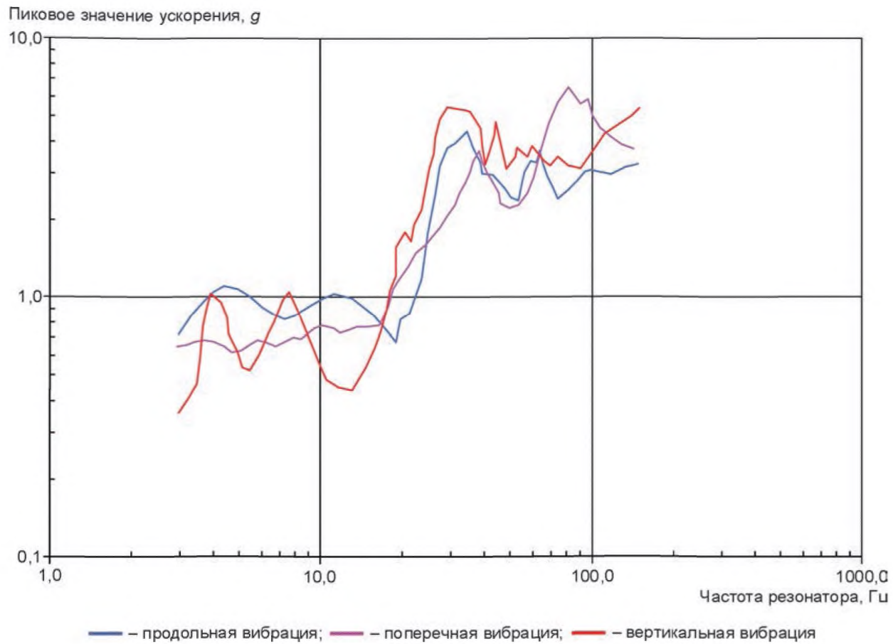
Рисунок 30 — Ударные спектры для повторяющихся событий, по данным [11] ( \zeta = 3\% , Q = 16,6 )
