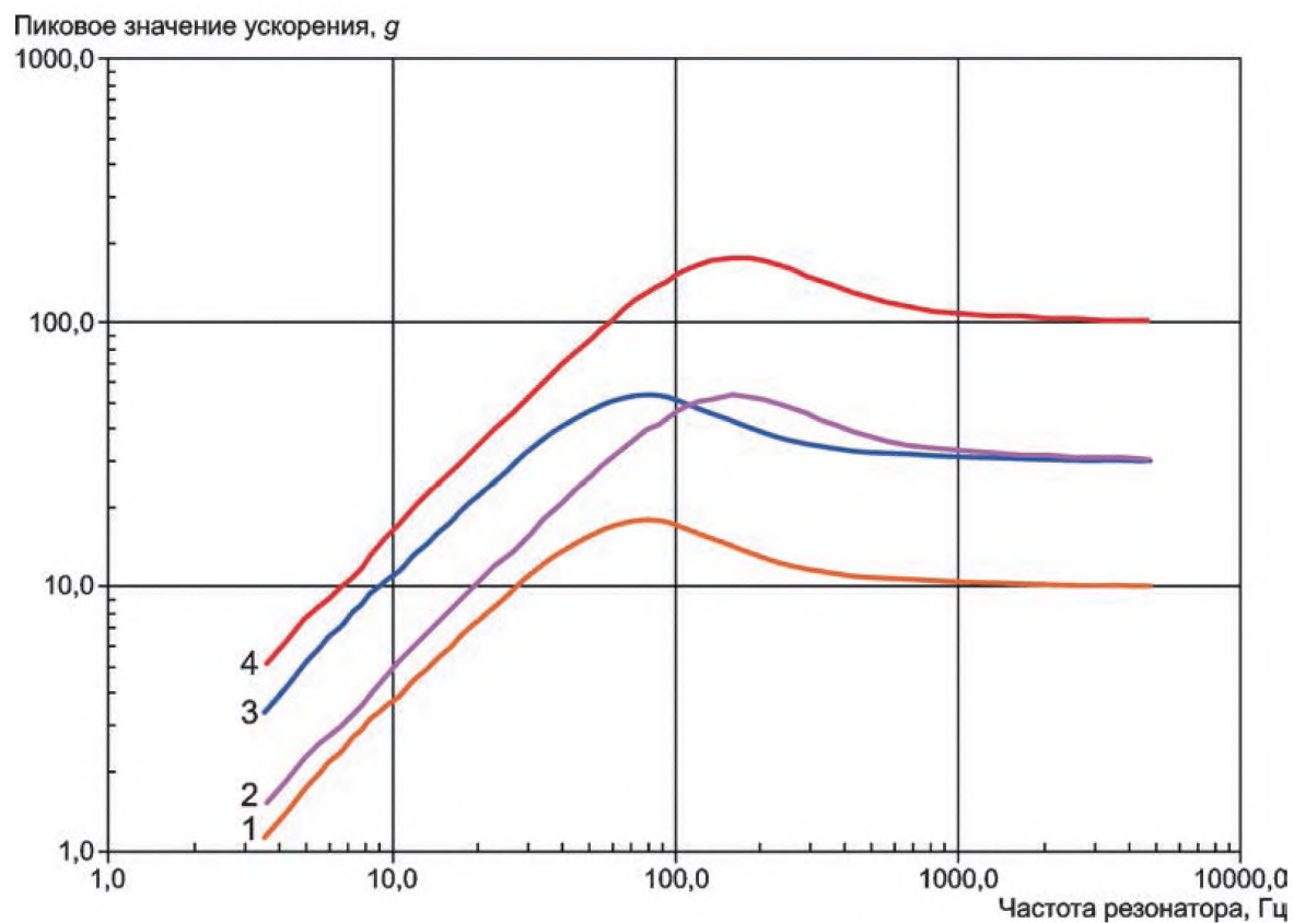
Рисунок 42 — Тестовые воздействия МЭК 60721-3-2:1997 (ударные спектры)
