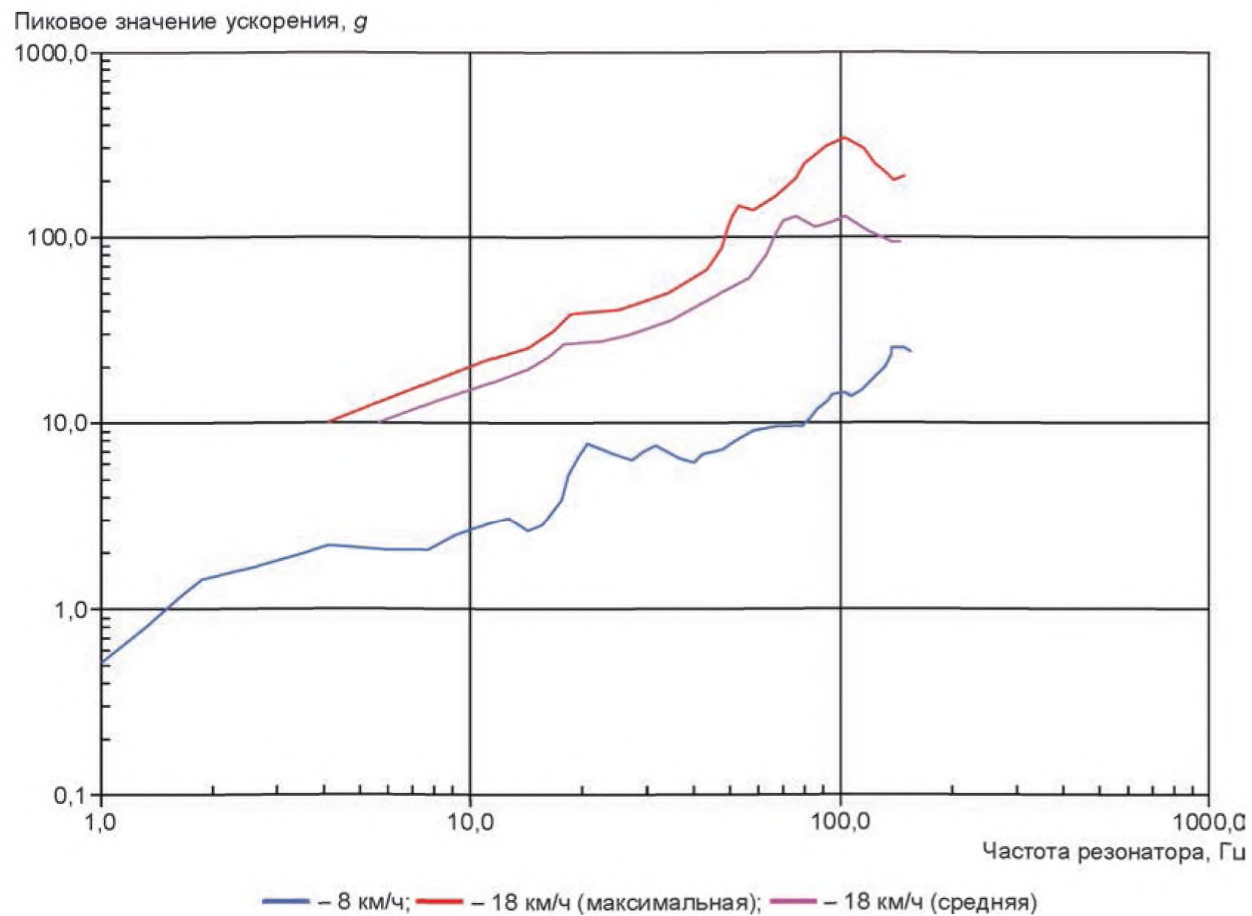
Рисунок 31 — Ударные спектры для случайных столкновений на разных скоростях, по данным [11] ( \zeta = 3\% , Q = 16,6 )
