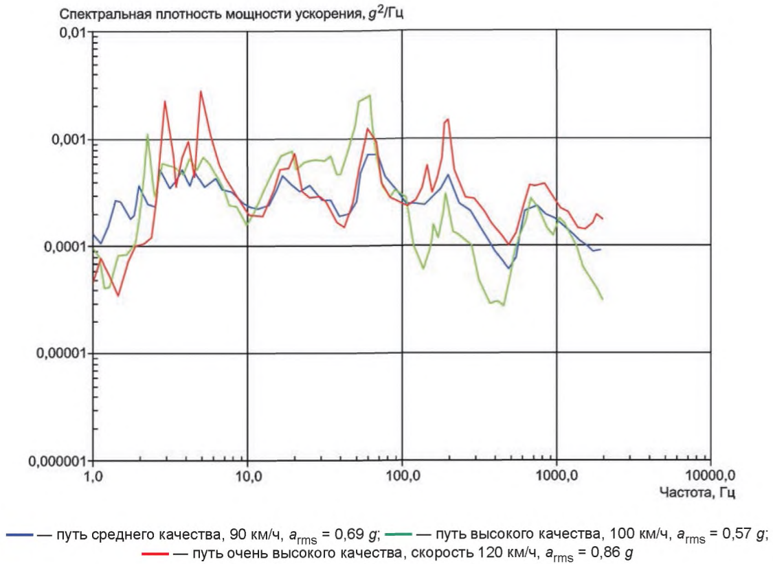
Рисунок 34 — Спектры вибрации в вертикальном направлении для вагонов Французской железнодорожной компании (SNCF) типов А, В и С, по данным [12]
