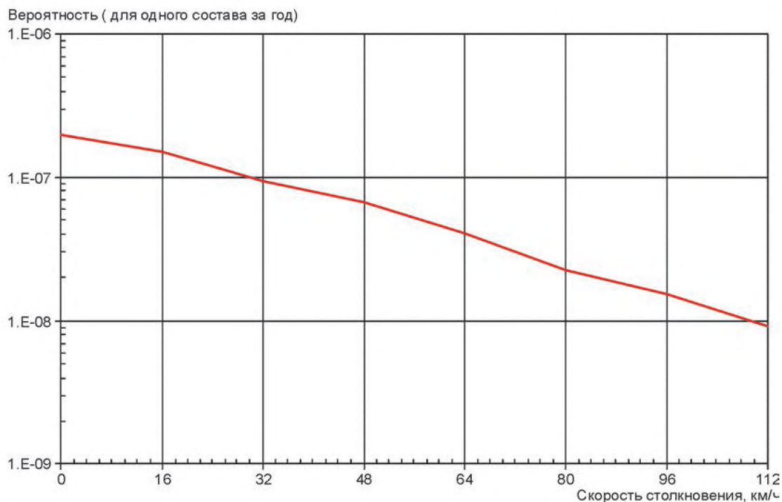
Рисунок 28 — Распределение по скоростям столкновения, по данным [10]
