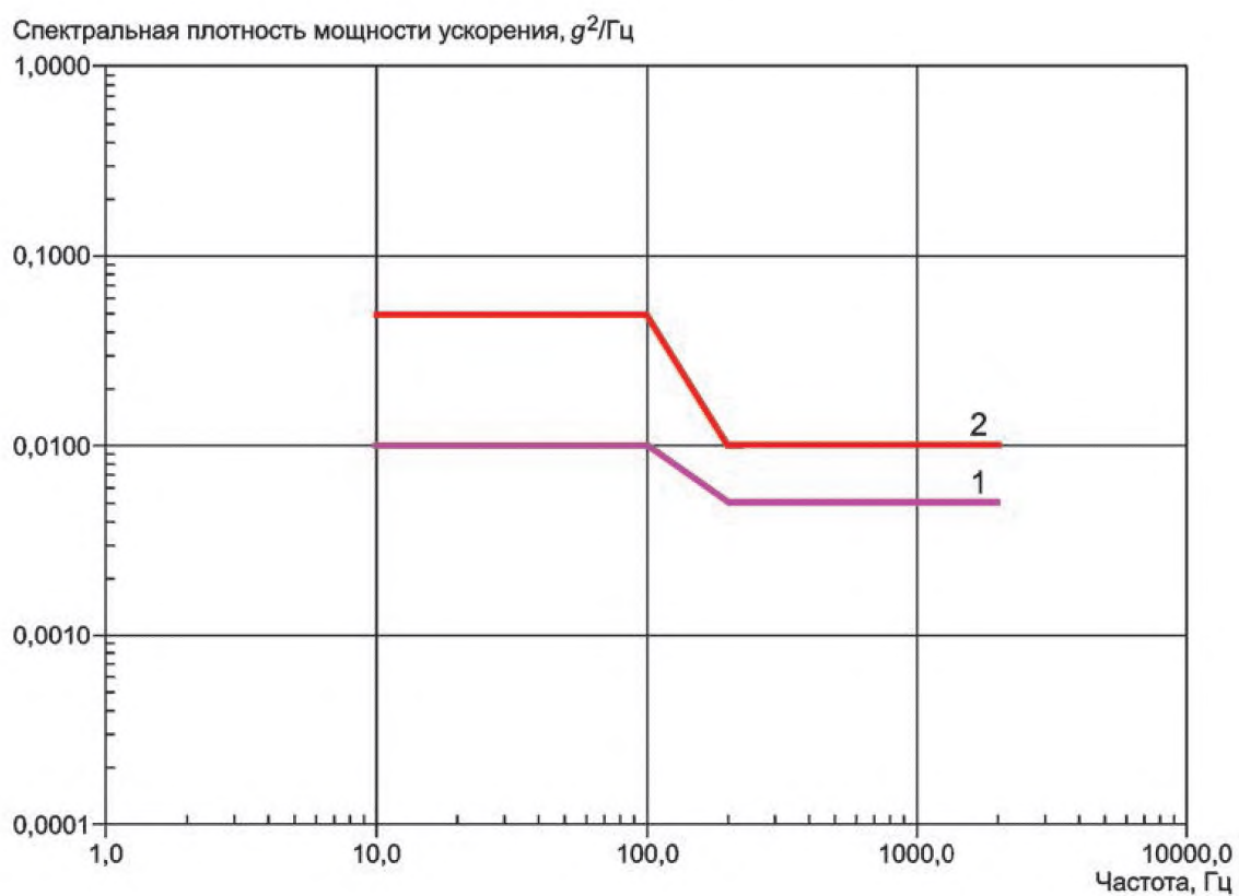
Рисунок 38 — Тестовые воздействия МЭК 60721-3-2:1997 (случайная вибрация)
