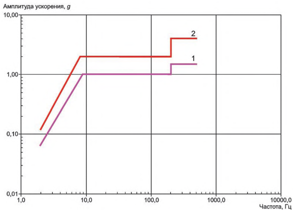
Рисунок 40 — Тестовые воздействия МЭК 60721-3-2:1997 (гармоническая вибрация)
