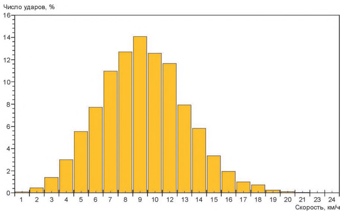
Рисунок 3 — Распределение скоростей столкновения (Британские железные дороги)
