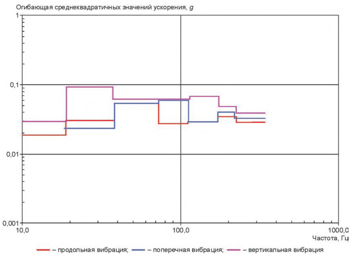
Рисунок 29 — Тестовые воздействия на вибрацию, по данным [11]
