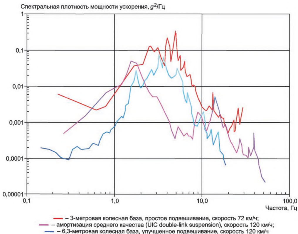
Рисунок 1 — Жесткость вибрации в вертикальном направлении (Британские железные дороги)
