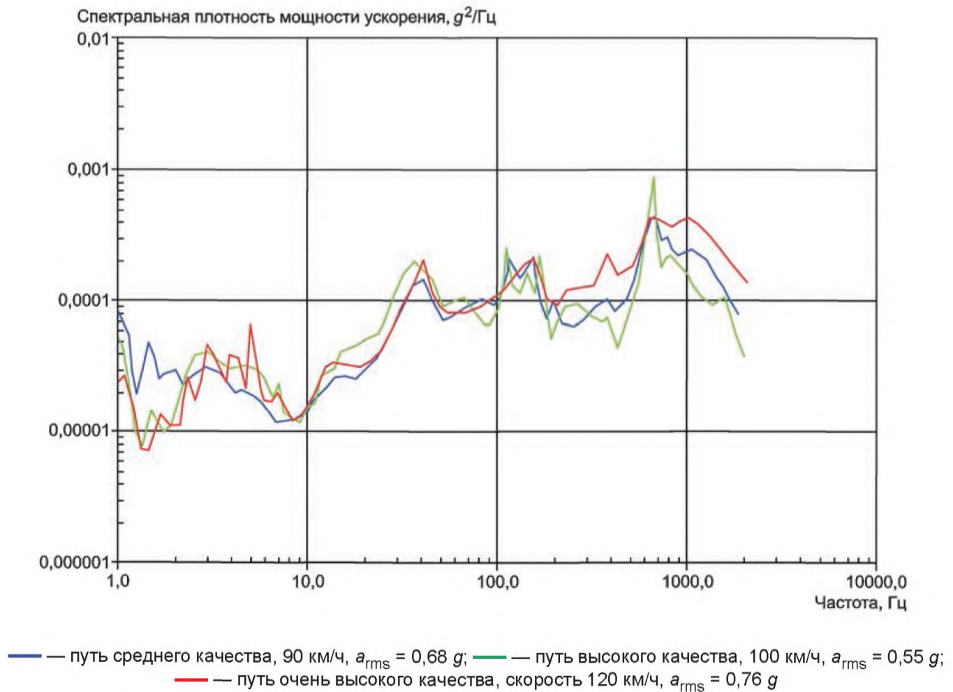
Рисунок 33 — Спектры вибрации в поперечном направлении для вагонов Французской железнодорожной компании (SNCF) типов А, В и С, по данным [12]
