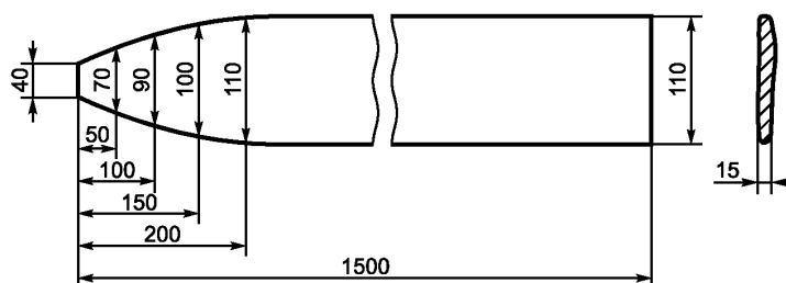
Рисунок 1 — Правилка А
