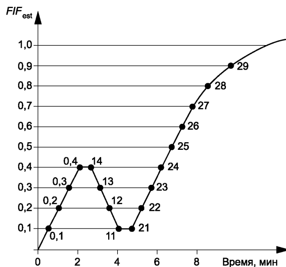
Рисунок 1 — Последовательность нагружения
