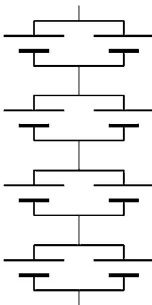
Рисунок А.4 — Структура 2P4S
