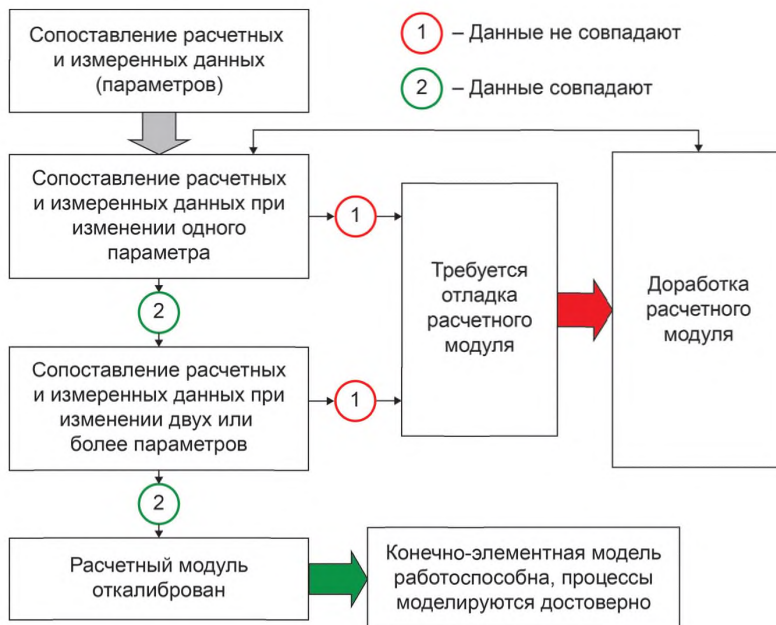
Рисунок 3 — Рекомендуемая блок-схема алгоритма калибровки КЭ модели
