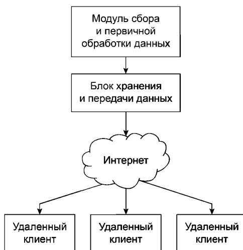
Рисунок 2 — Схема организации обмена данными СМНМЭП
