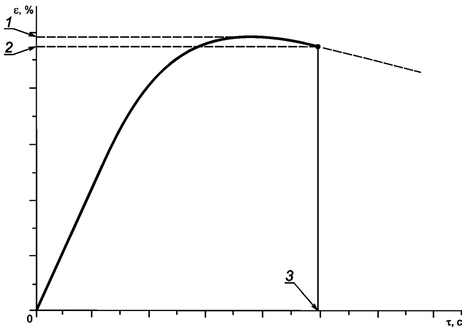
Рисунок 1 — Схема определения момента начала спада на диаграмме «деформация — время» при нагреве
