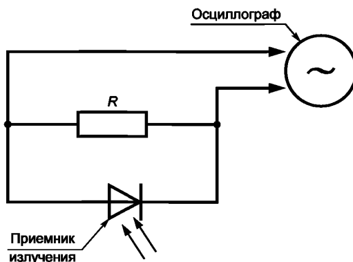
Рисунок 1 — Схема измерения пульсаций освещенности с помощью осциллографа
