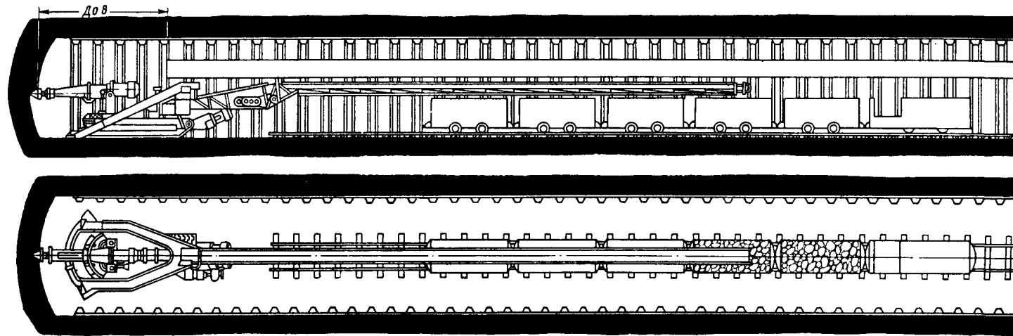
Схема обмена вагонеток
