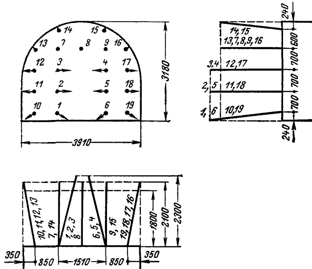
Схема расположения шпуров
