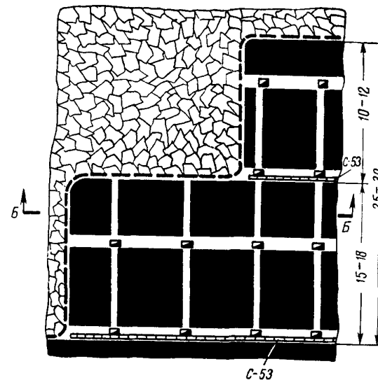
Схема очистного забоя
