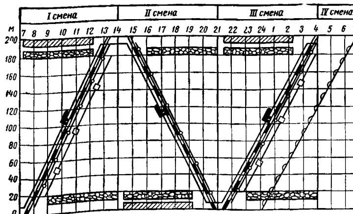
График выходов
