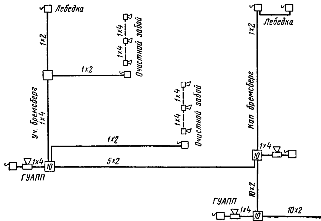
Рис. 43. Схема связи и сигнализации применительно к технологическим схемам очистных работ № 33 и 34
