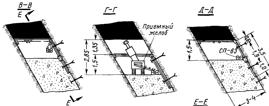
Конструкция раздвижного верхняка
