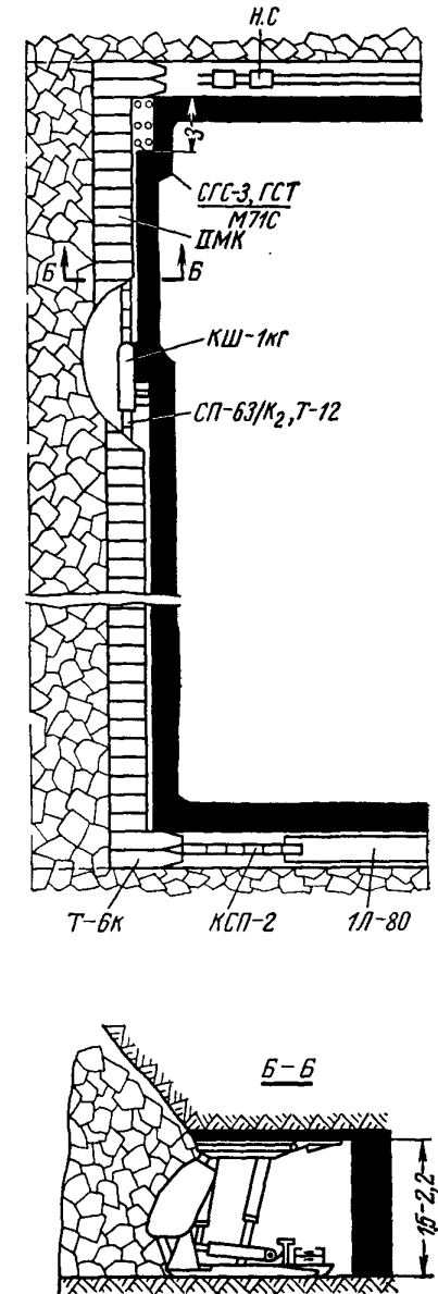
Схема очистного забоя
