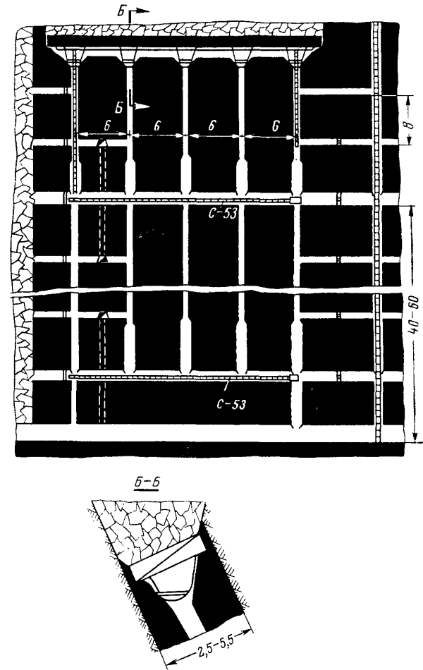
Схема очистного забоя
