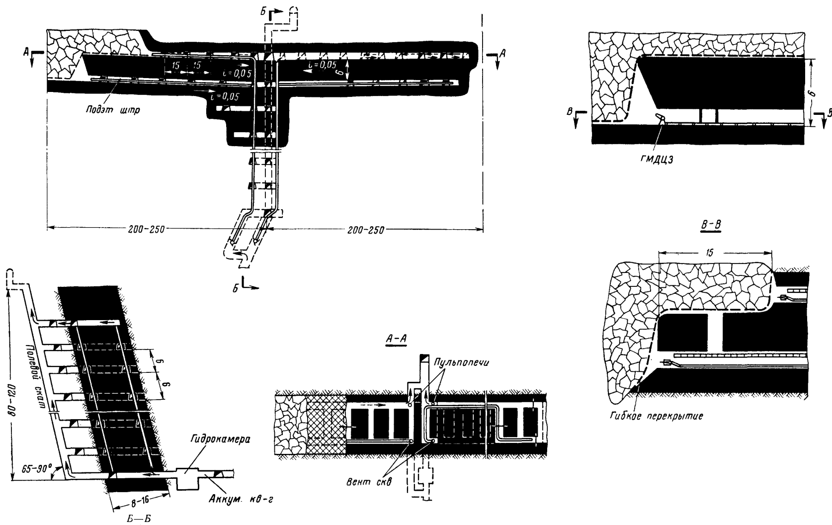
Схема очистного забоя
