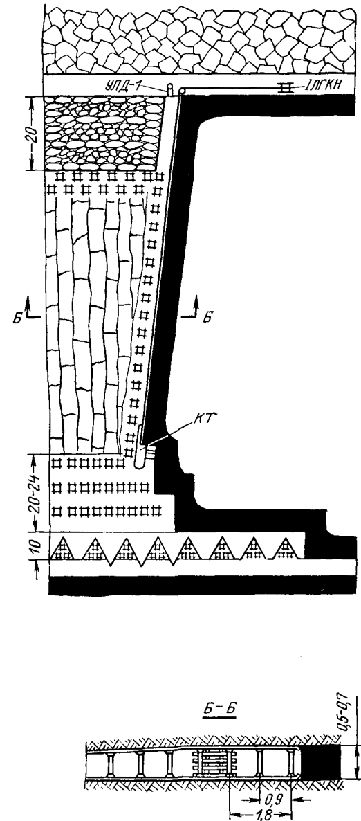
Схема очистного забоя
