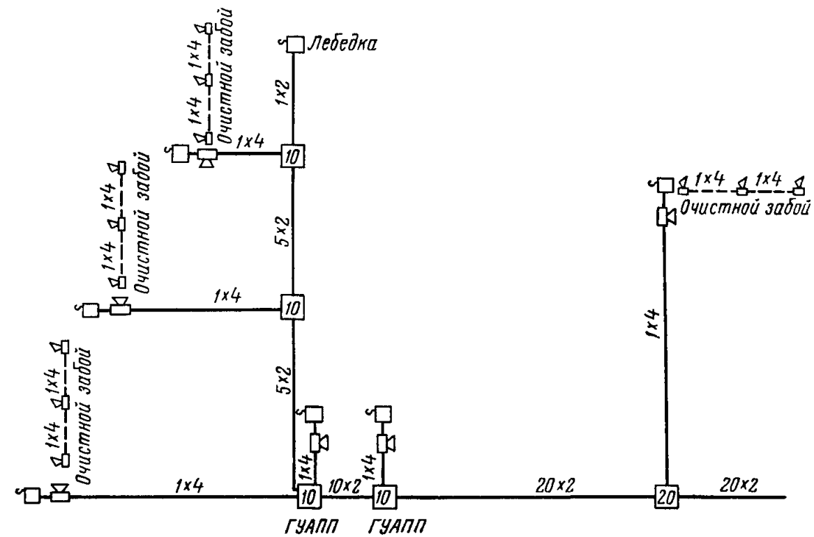
Рис. 47. Схема связи и сигнализации применительно к технологическим схемам очистных работ № 51 и 52
