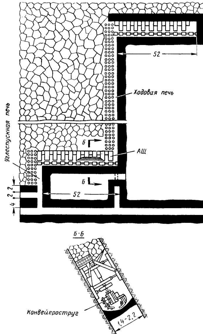
Схема очистного забоя
