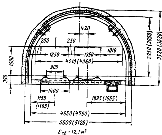
Характеристика выработки
