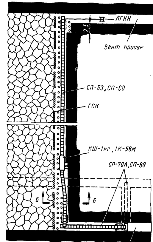
Схема очистного забоя
