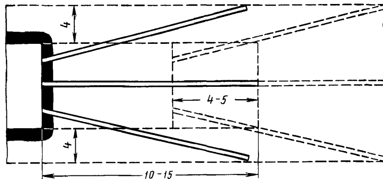
Рис. 6. Схема расположения опережающих скважин
