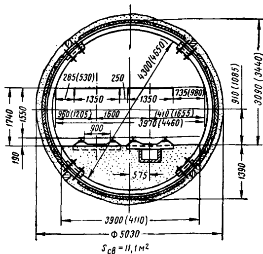
Характеристика выработки
