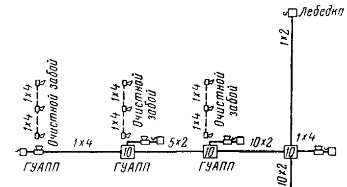
Рис. 46. Схема связи и сигнализации применительно к технологическим схемам очистных работ № 48—50
