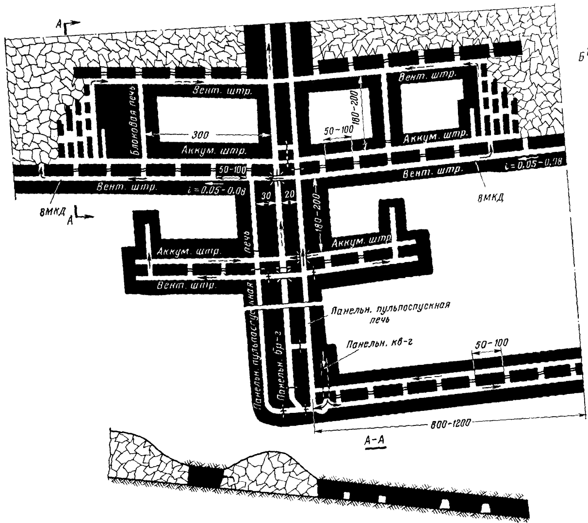
Схема 37
