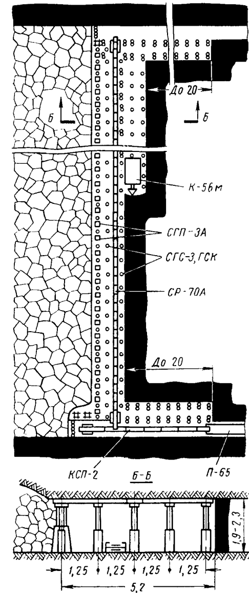
Схема очистного забоя
