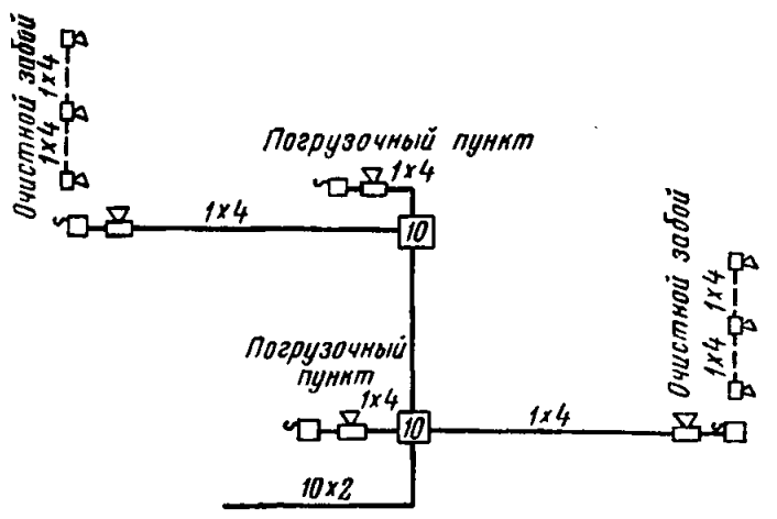
Рис. 38. Схема связи и сигнализации применительно к технологическим схемам очистных работ № 21—23
