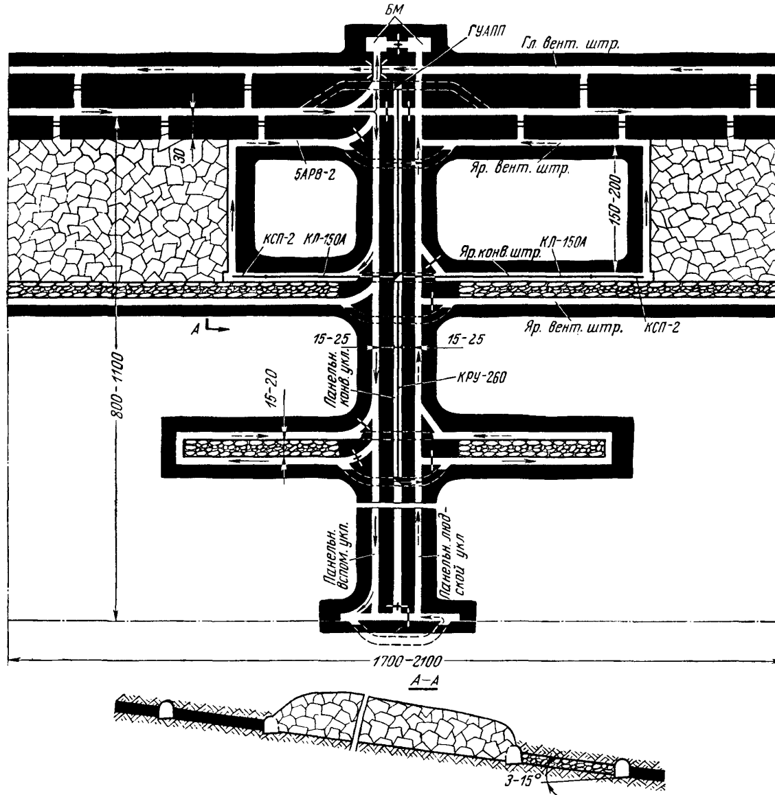
ТЕХНОЛОГИЯ ОЧИСТНЫХ РАБОТ С КОМБАЙНАМИ МК, 1К-101 Схема подготовки и система разработки
