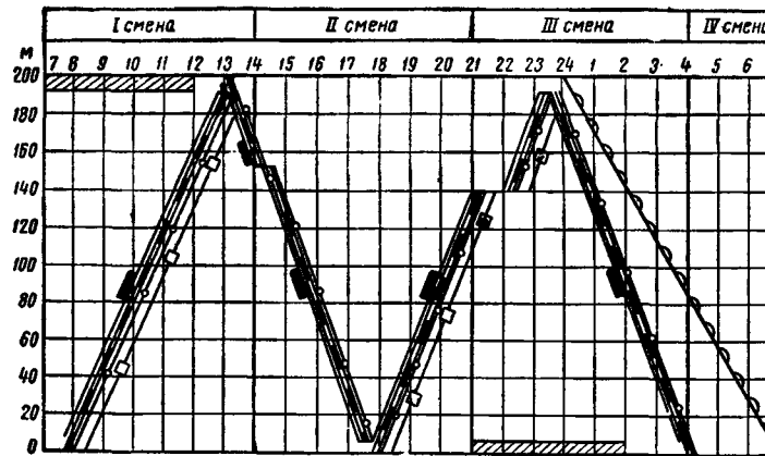
Планограмма работ
