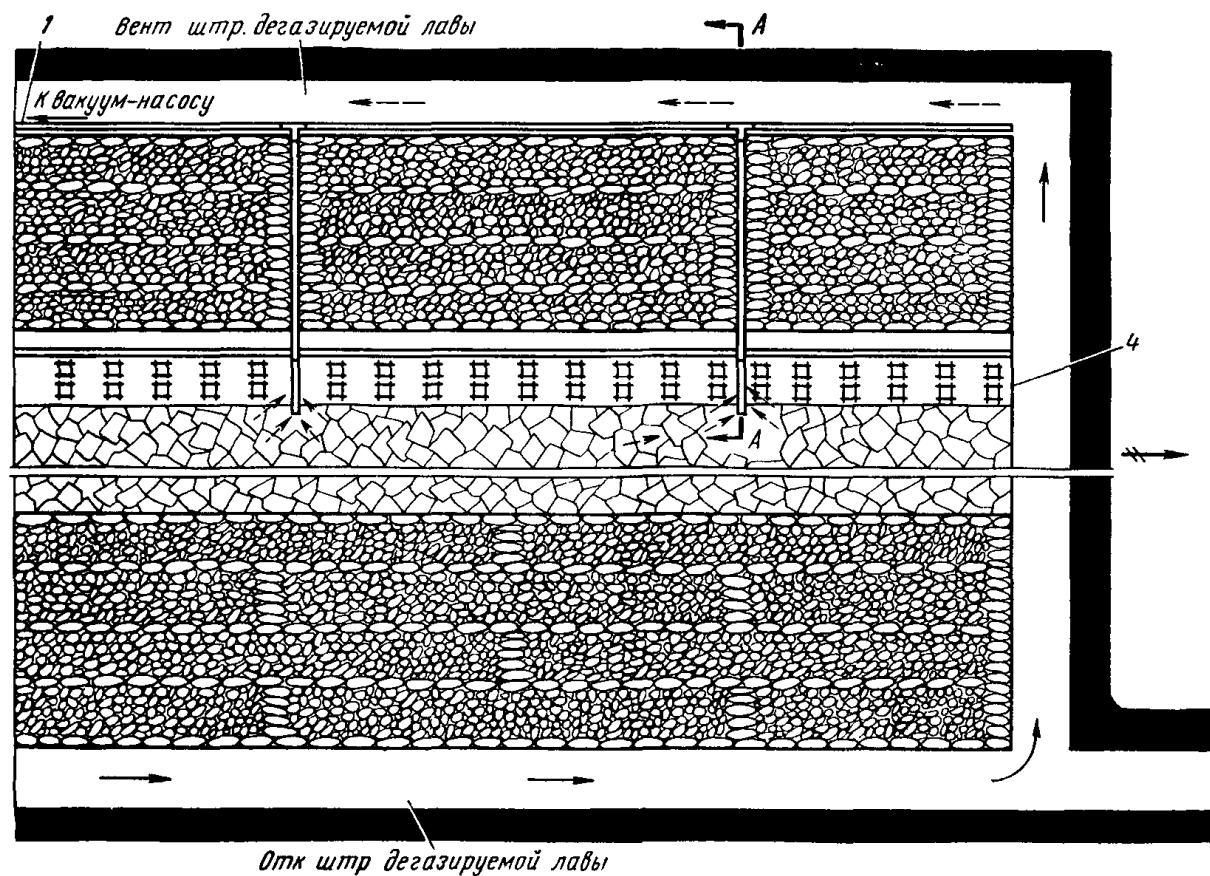
Рис. 10. Схема дегазации подрабатываемых спутников применительно к технологическим схемам очистных работ № 5, 17, 19, 26, 27 и 30
