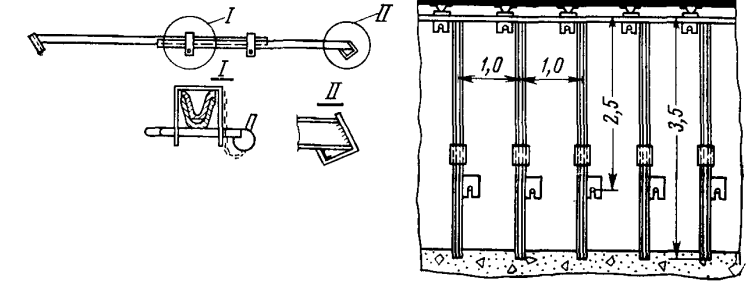
Конструкция раздвижного верхняка
