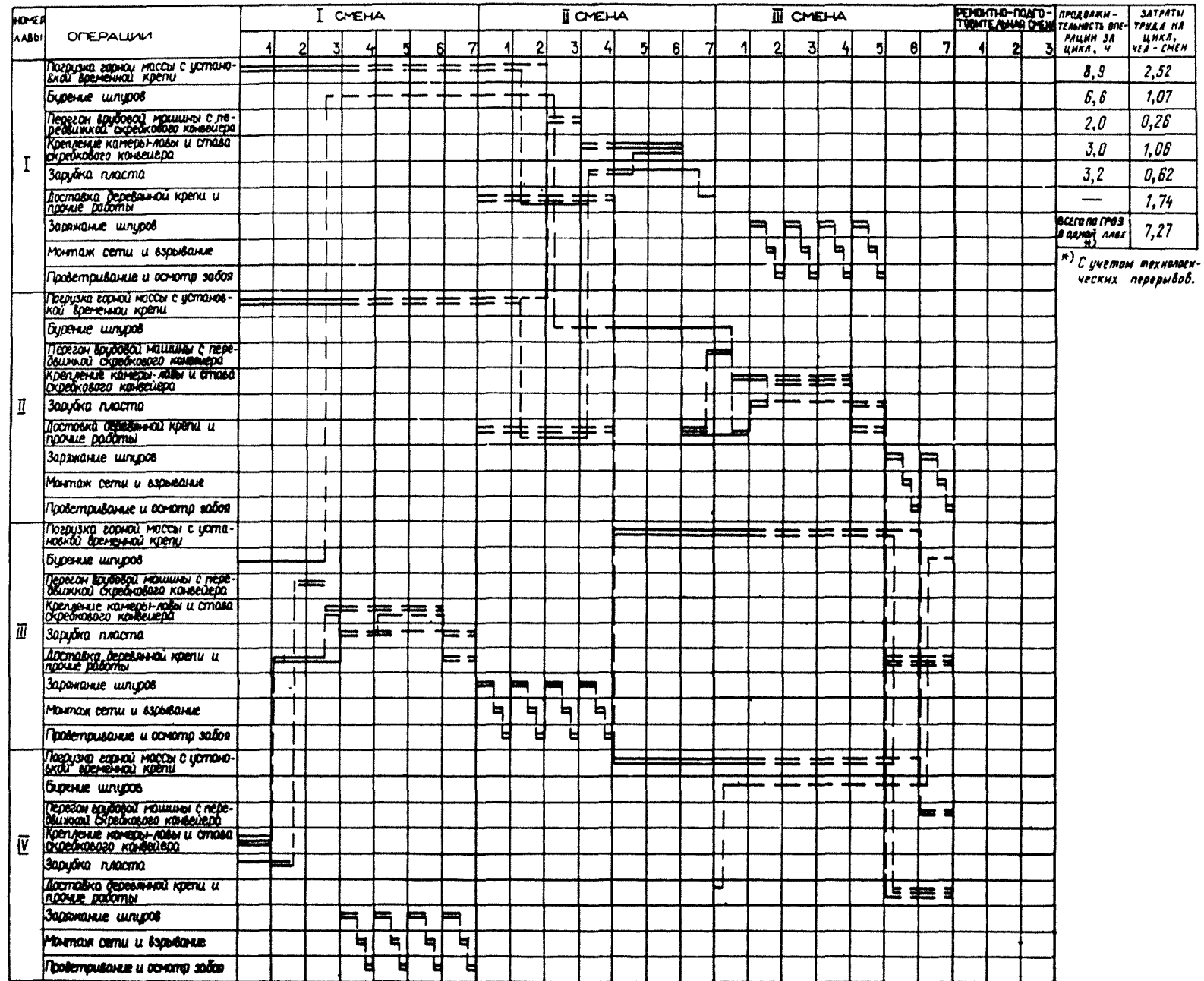
Рис. 13.3. График организации работ в счетверенных камерах-лавах с применением бурового станка БУА-30
