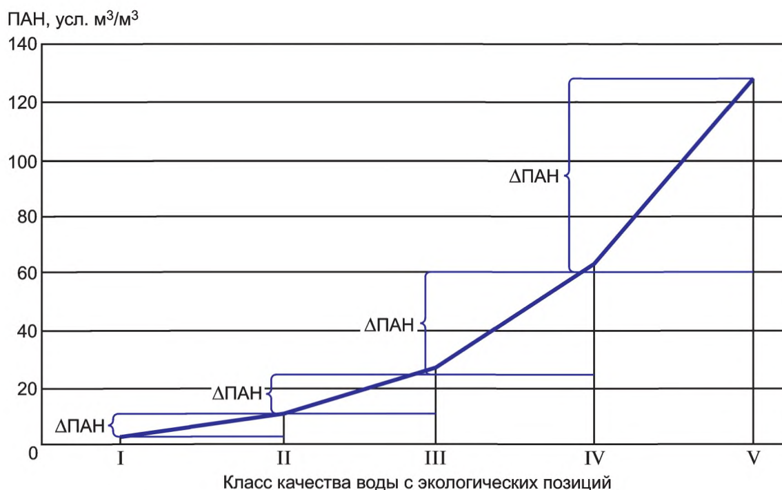
Рисунок Б.1 — Изменение значения ПАН при изменении класса качества воды
