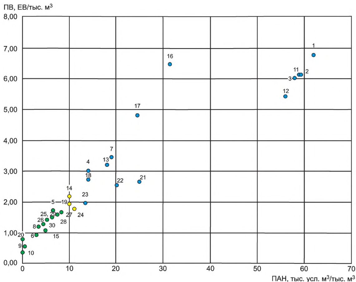
Рисунок Г.1 — Точечная диаграмма зависимости ПАН от ПВ для очищенных хозяйственно-бытовых сточных вод
