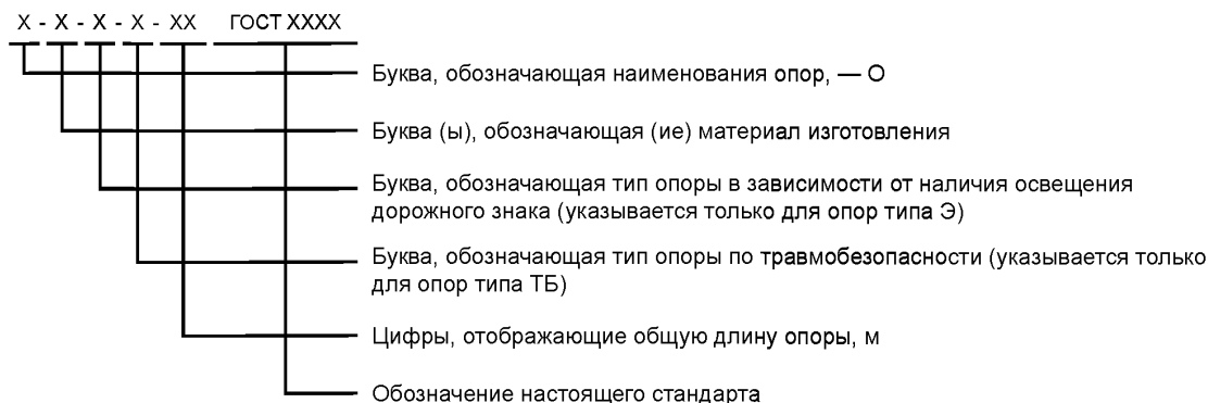
Рисунок 1 — Схема условного обозначения опор
