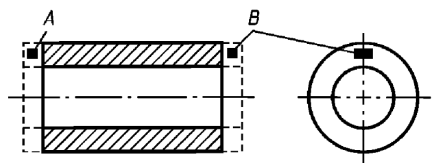
Рис. П11.2.5.4.5. Места отбора проб из поковок муфт и обечаек
