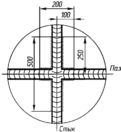
Рис. 8.1.12-2. Контроль участков паза с каждой стороны стыка
