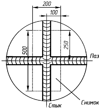
Рис. 8.1.12-1. Расположение снимка при контроле сварных швов
