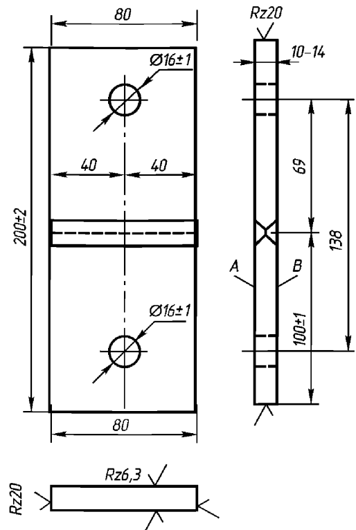
Рис. П6.2. Образец для испытания на стойкость против коррозии
