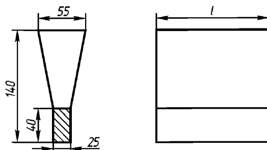
Рис. П11.2.9.1-3. Размеры проб V-образной формы
