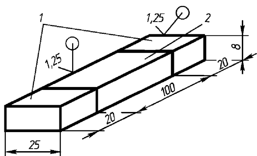
Рис. П9.2.4. Стальная шлифованная пластина, собранная вместе с выводными планками:
