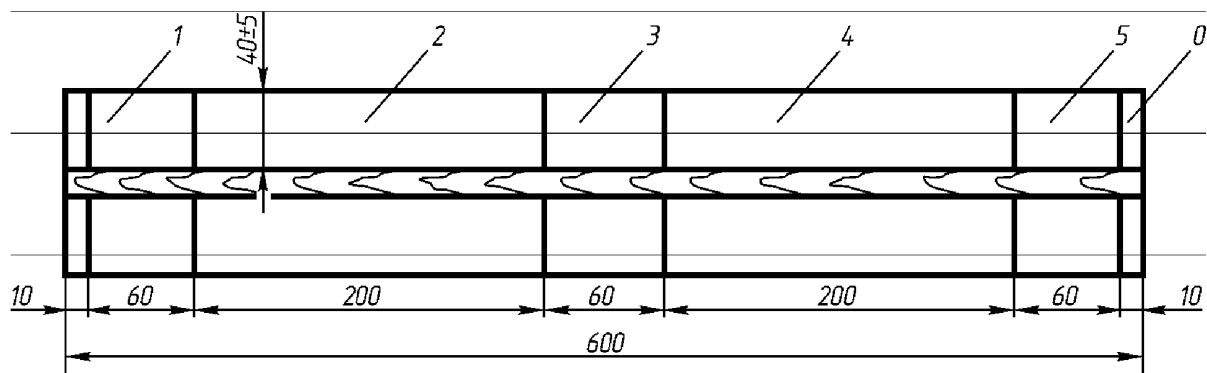
Рис. П7.8.2-1. Схема вырезки заготовок для макрошлифов из стыкового соединения пробы: 0 — отход; 1, 3, 5 — заготовки для поперечных макрошлифов и круглых разрывных образцов; 2, 4 — заготовки для продольных макрошлифов
