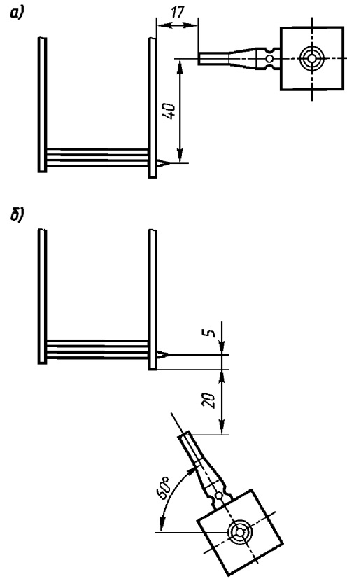
Рис. П4.4-2. Положение горелки относительно образца ткани
