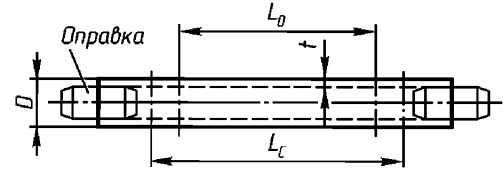
Рис. П10.2.3-4. Образец для испытаний на растяжение в виде участка трубы
