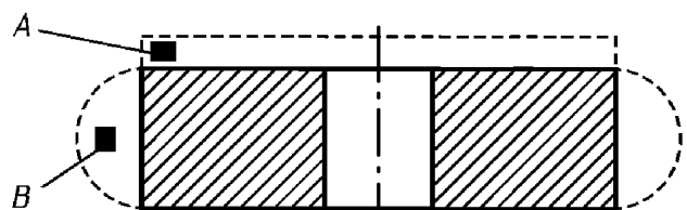
Рис. П11.2.5.4.3. Места отбора проб из поковок зубчатых колес
