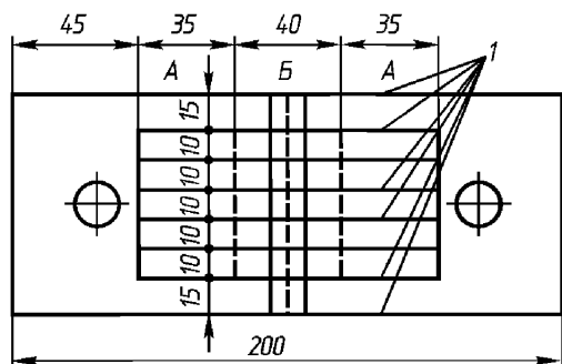
Рис. Пб.5. Схема профилометрирования сварного образца:
