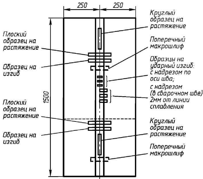
Рис. П12.6.2-1. Проба для испытания сварочных материалов для дуговой сварки в защитном газе
