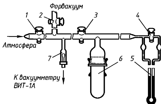
Рис. П9.6.1. Прибор для определения содержания диффузионно-подвижного водорода:
