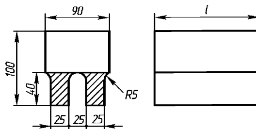
Рис. П11.2.9.1-2. Размеры проб U-образной формы типа IIb
