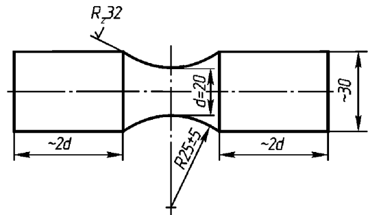
Рис. П10.2.4 Цилиндрический образец для испытаний на растяжение серого чугуна
