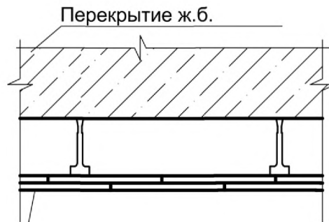
Подвесные потолки для повышения пределов огнестойкости перекрытий [п.5.2.6 СП 2.13130]
