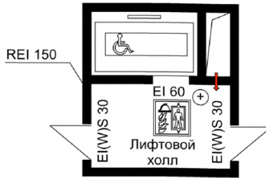
Схемы размещения лифтов для пожарных
