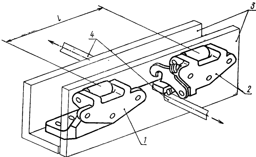
Схема приложения продольной нагрузки
