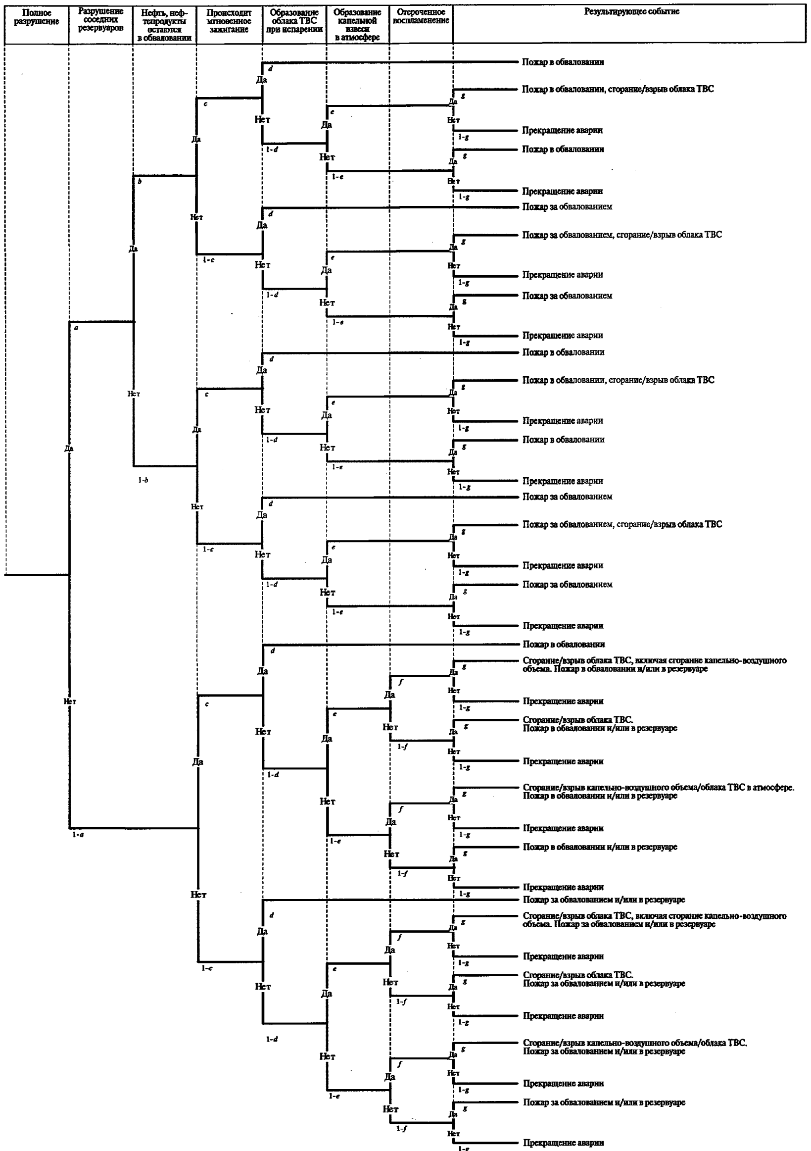
Рис. 5. Дерево событий разрушения (перелива) наземного резервуара (сценарий А 1 )
