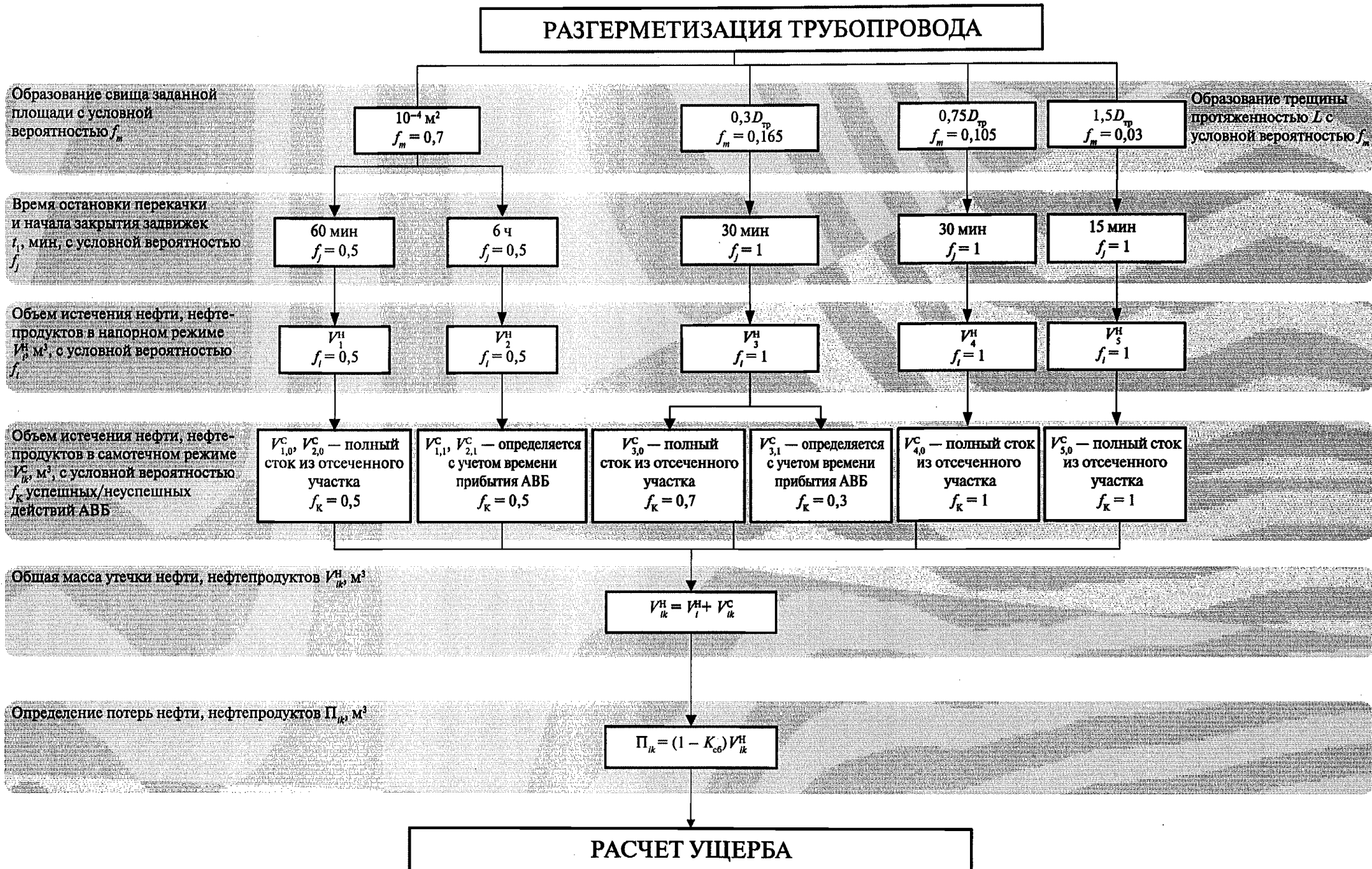
Рис. 4. Алгоритм расчета аварийных утечек нефти, нефтепродуктов из ОПО МН и МНПП с учетом типового времени обнаружения утечки, остановки насосов и начала перекрытия потока трубопроводной арматурой
