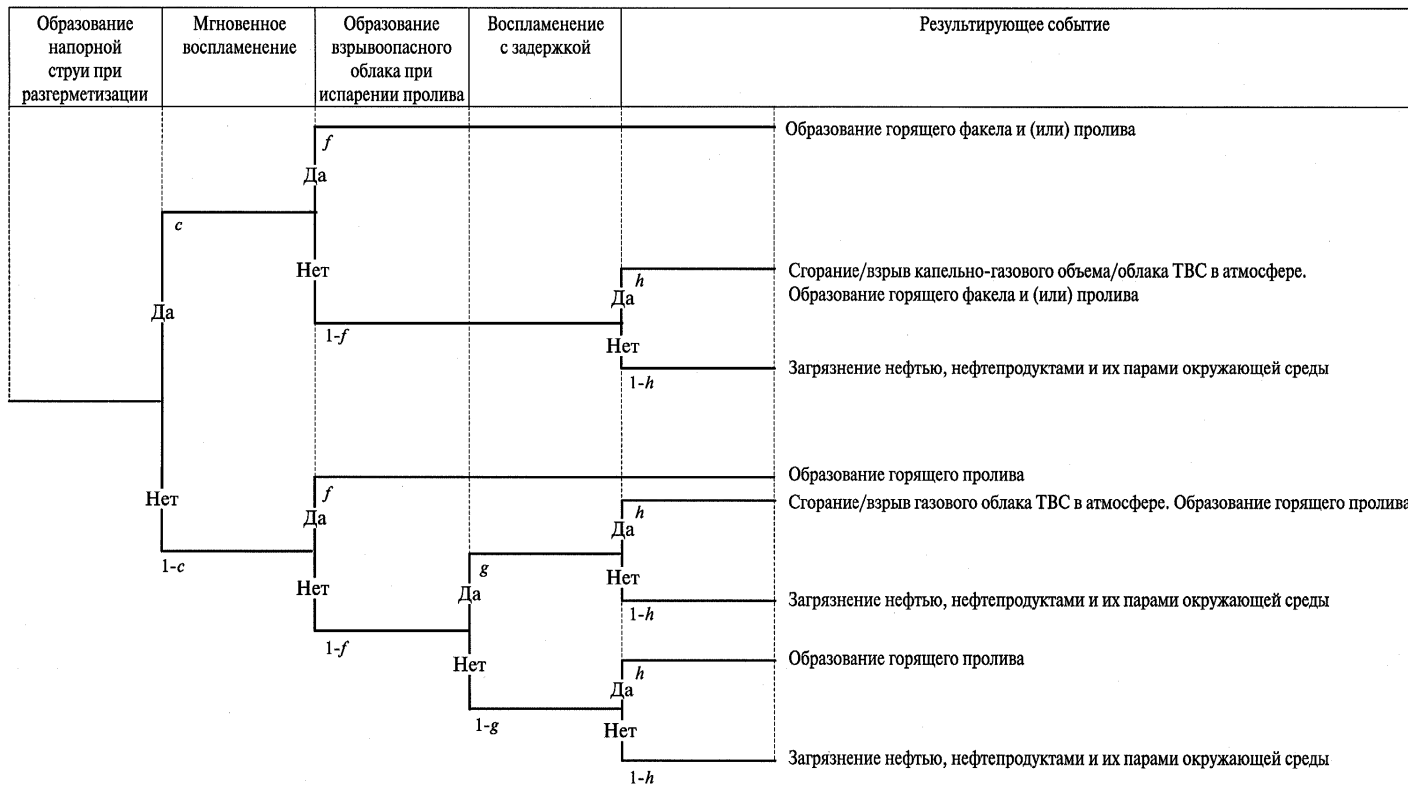
Рис. 3. Дерево событий при разгерметизации подземного участка ЛЧ ОПО МН и МНПП
