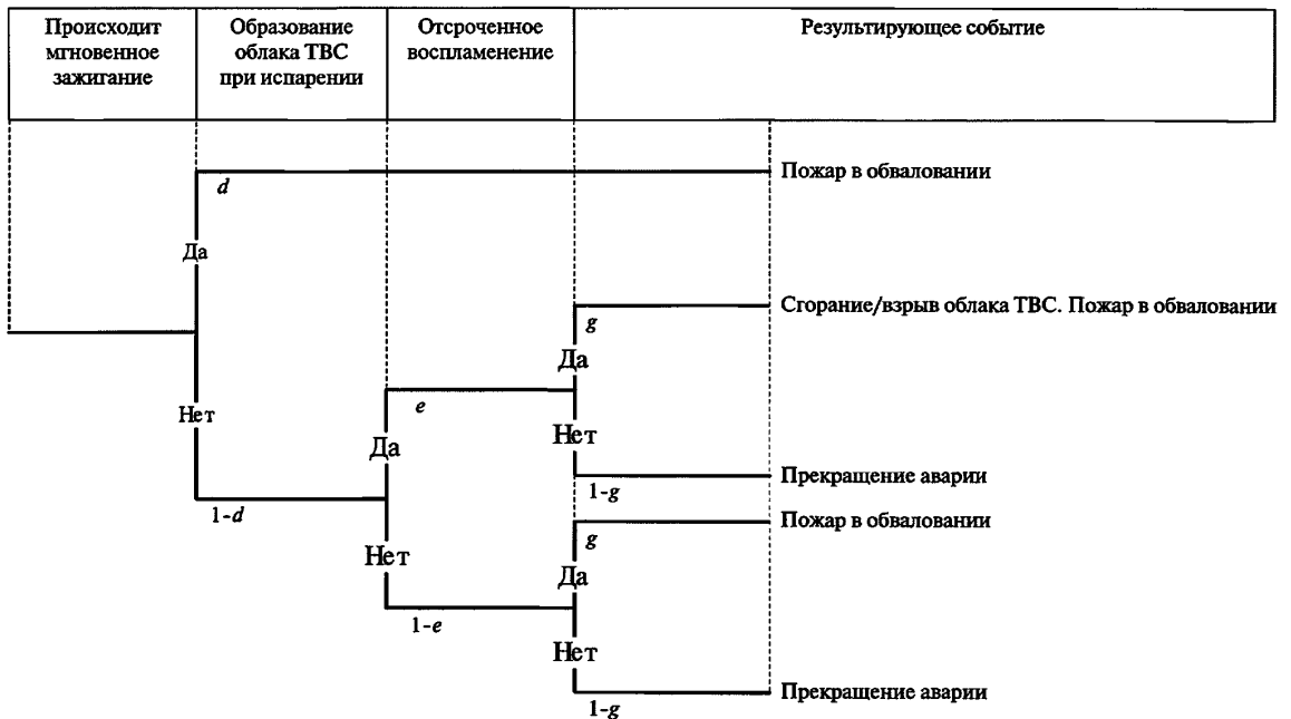
Рис. 8. Дерево событий разрушения (перелива) подземного резервуара (сценарий A 4 )
