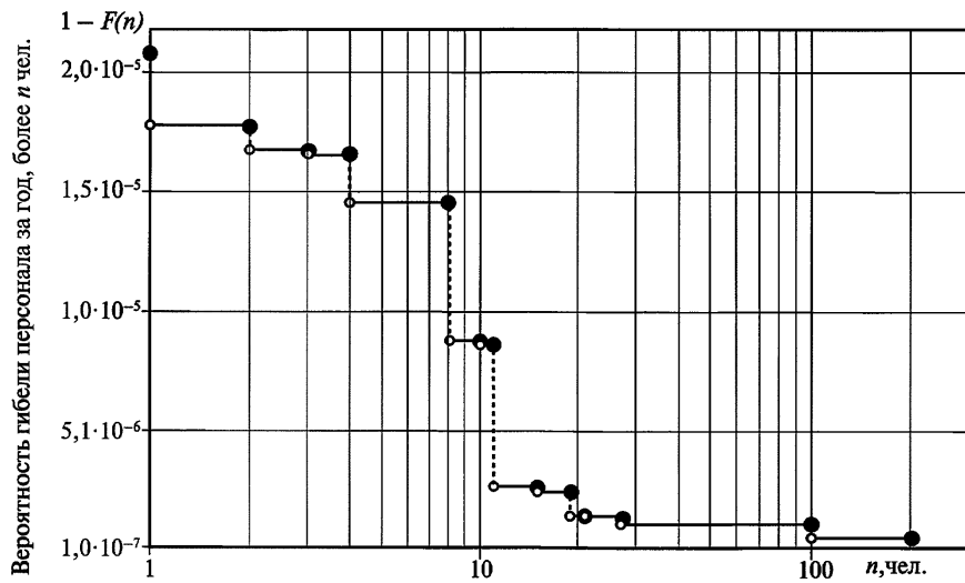
Рис. 2. Пример интегральной функции распределения числа погибших при аварии на резервуарном парке ( F/N -кривая)
