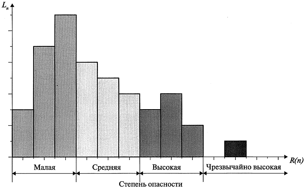
Рис. 16. Иллюстрация формы представления распределения суммарной длины участков L_s трассы по показателю риска аварий R
