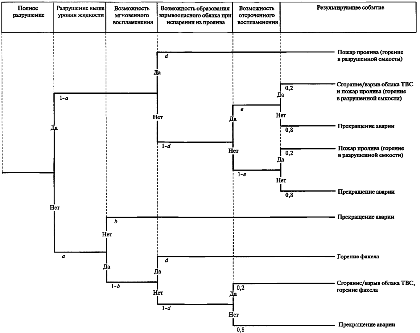
Рис. 12. Дерево событий при разрушении подземной емкости под давлением (сценарий А 8 )
