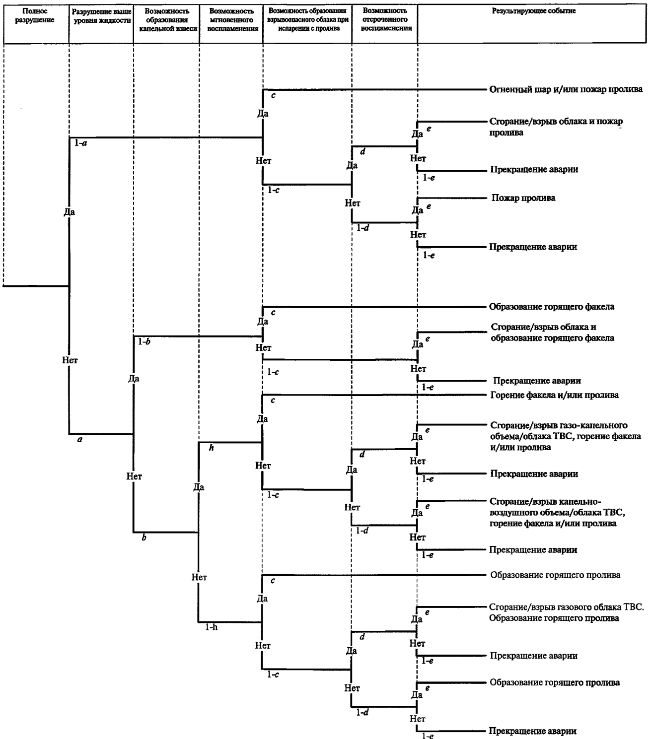
Рис. 11. Дерево событий при разрушении емкости под давлением (сценарий А 7 )
