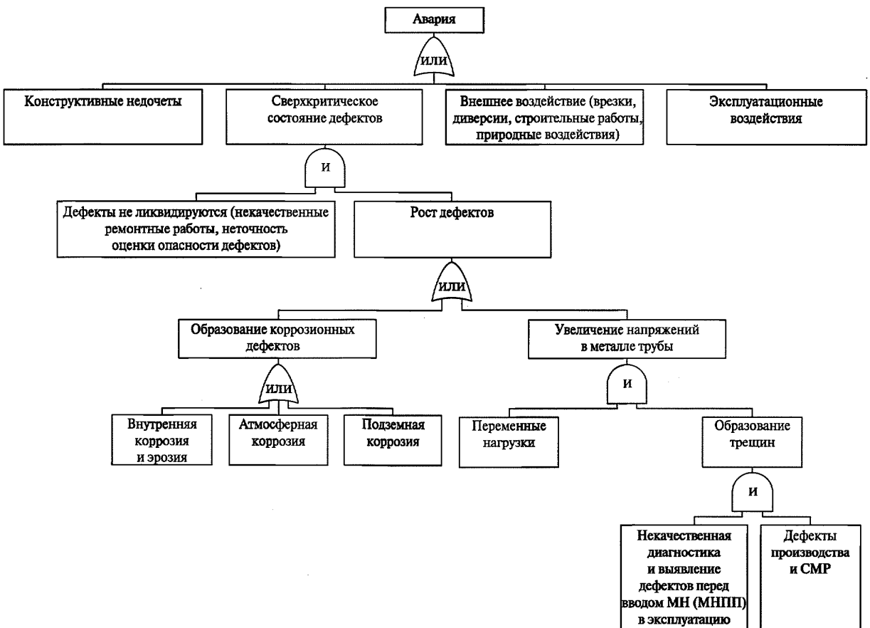
Рис. 2. Дерево отказов для аварий на ЛЧ ОПО МН и МНПП
