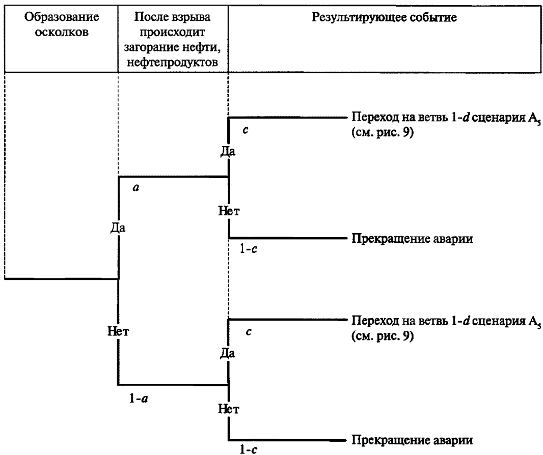
Рис. 10. Дерево событий при взрыве внутри подземного резервуара (типа ЖБР) (сценарий A 6 )
