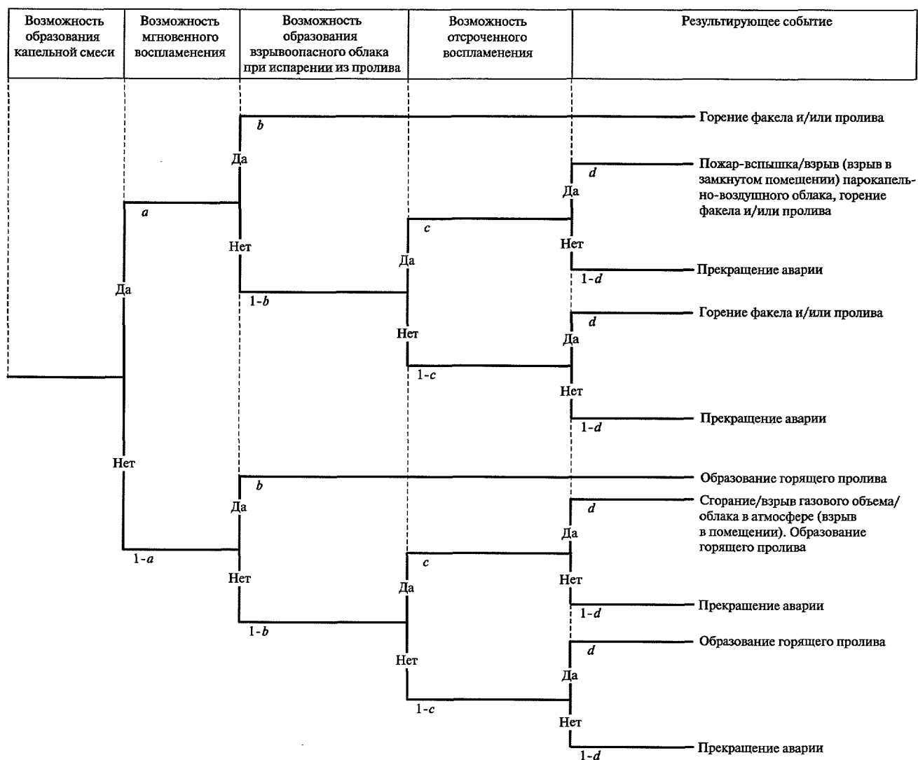
Рис. 13. Дерево событий при аварии в насосных (сценарий А 9 )
