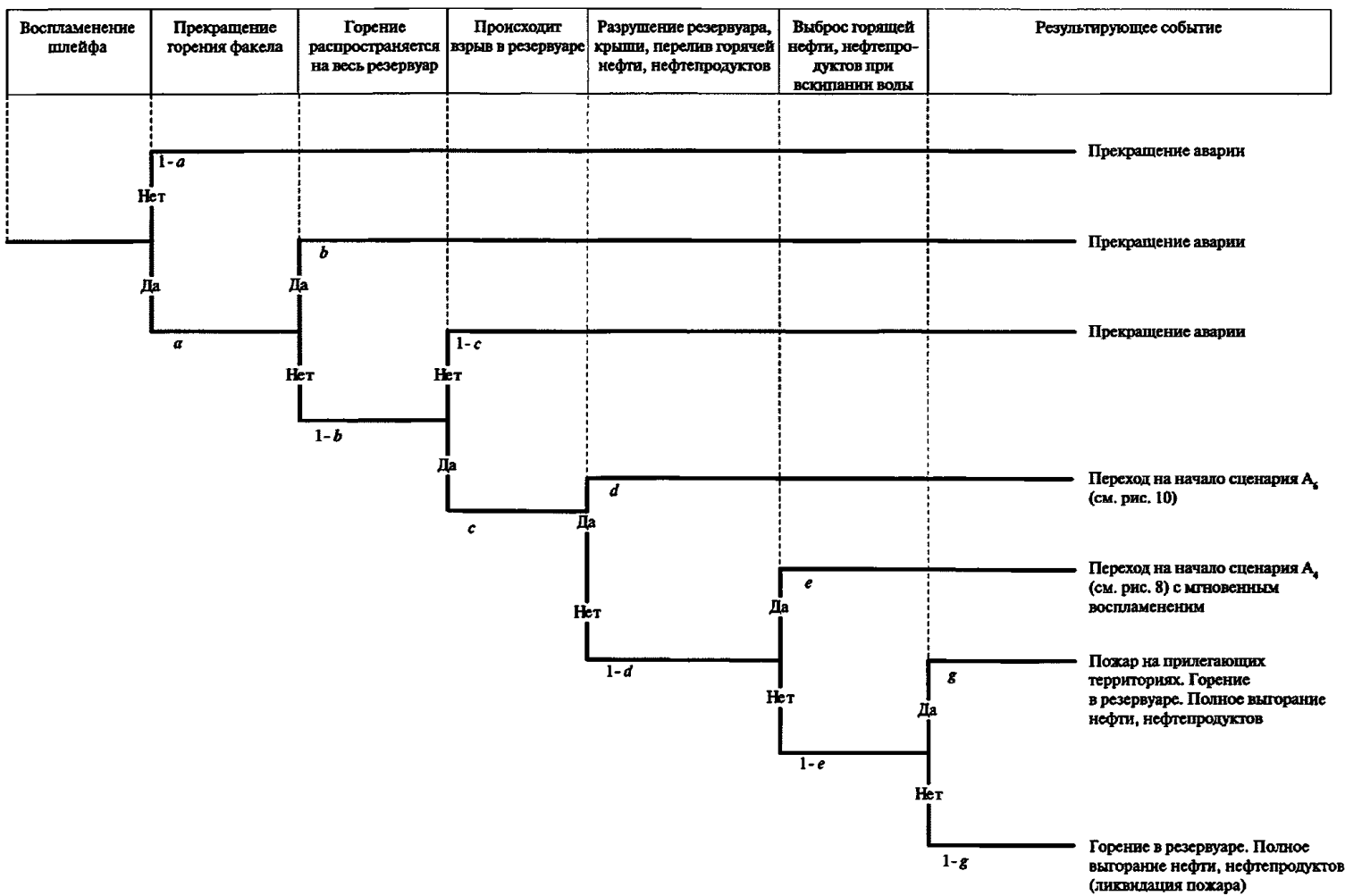
Рис. 9. Дерево событий при выходе газовой фазы из подземного резервуара (типа ЖБР) (сценарий A 2 )
