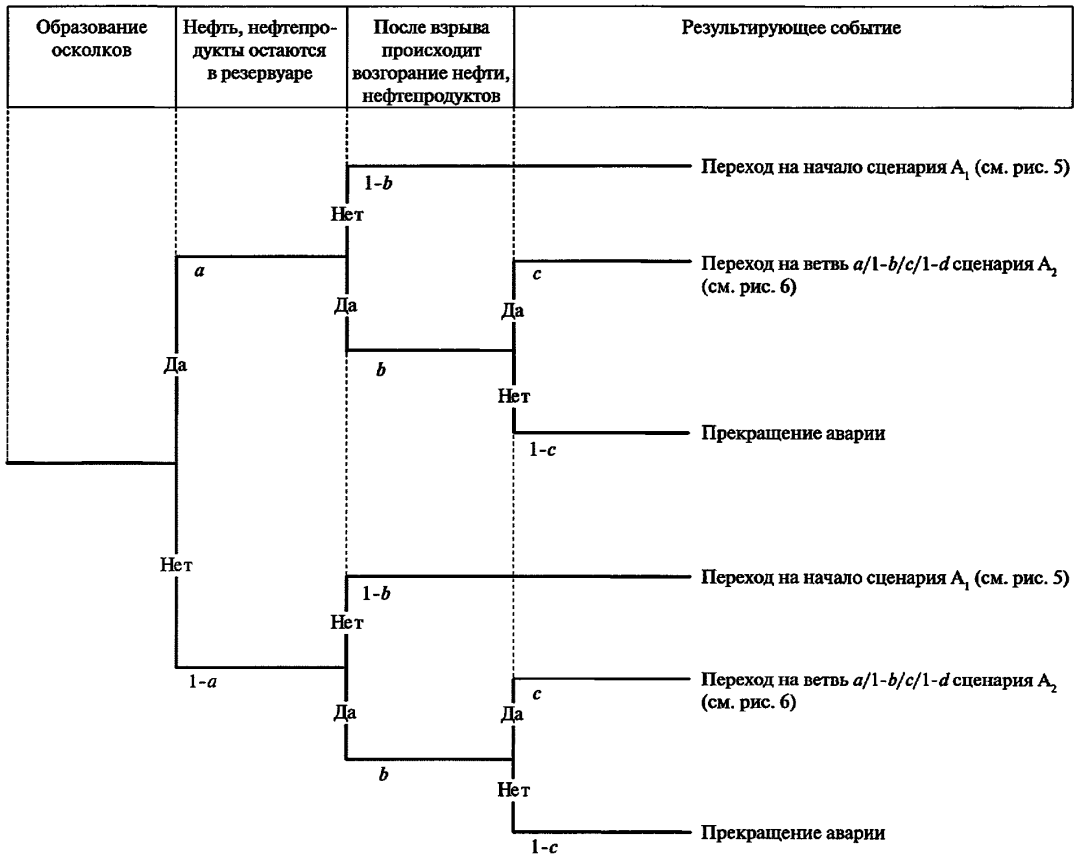
Рис. 7. Дерево событий при взрыве внутри наземного резервуара (сценарий A 3 )
