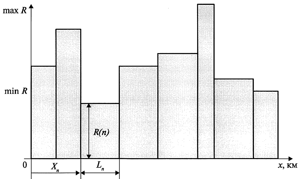
Рис. 15. Общий вид распределения показателя риска R(n) вдоль трассы ОПО МН и МНПП
