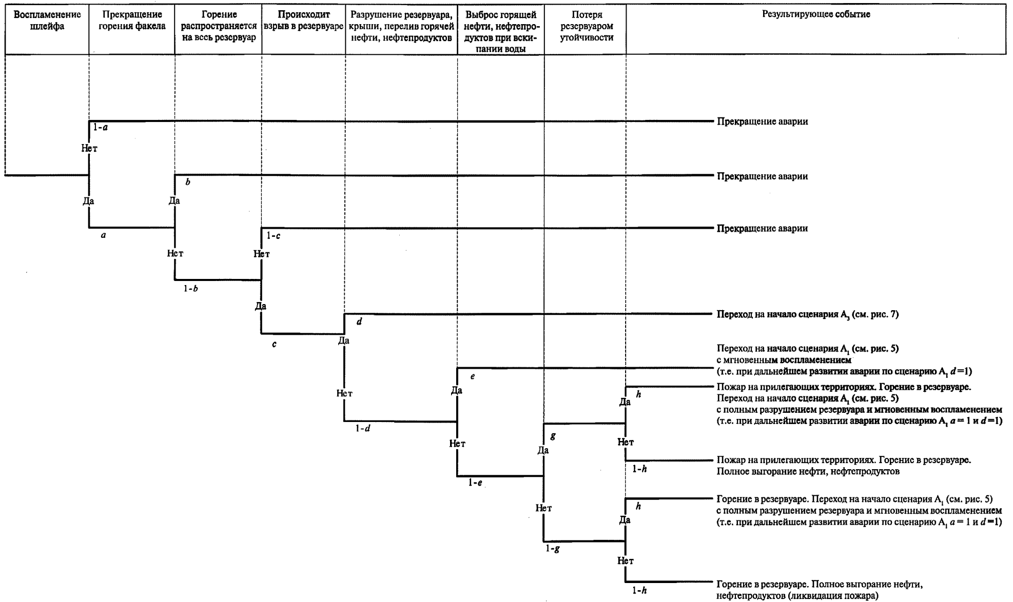
Рис. 6. Дерево событий при выходе газовой фазы с наземного резервуара (сценарий A 2 )
