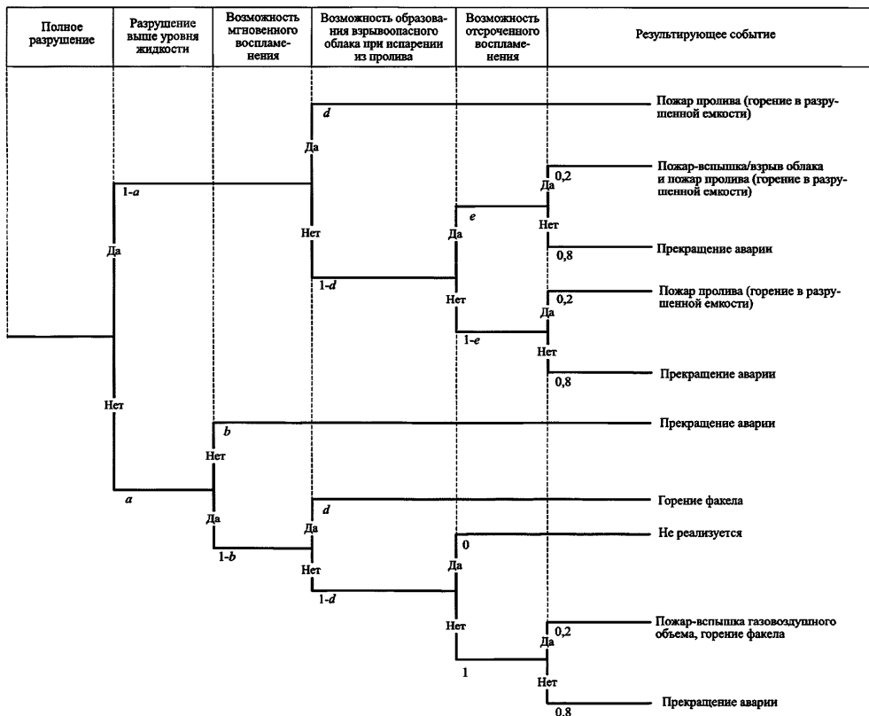
Рис. 7. Дерево событий при разрушении емкости под давлением (сценарий A_7 )
