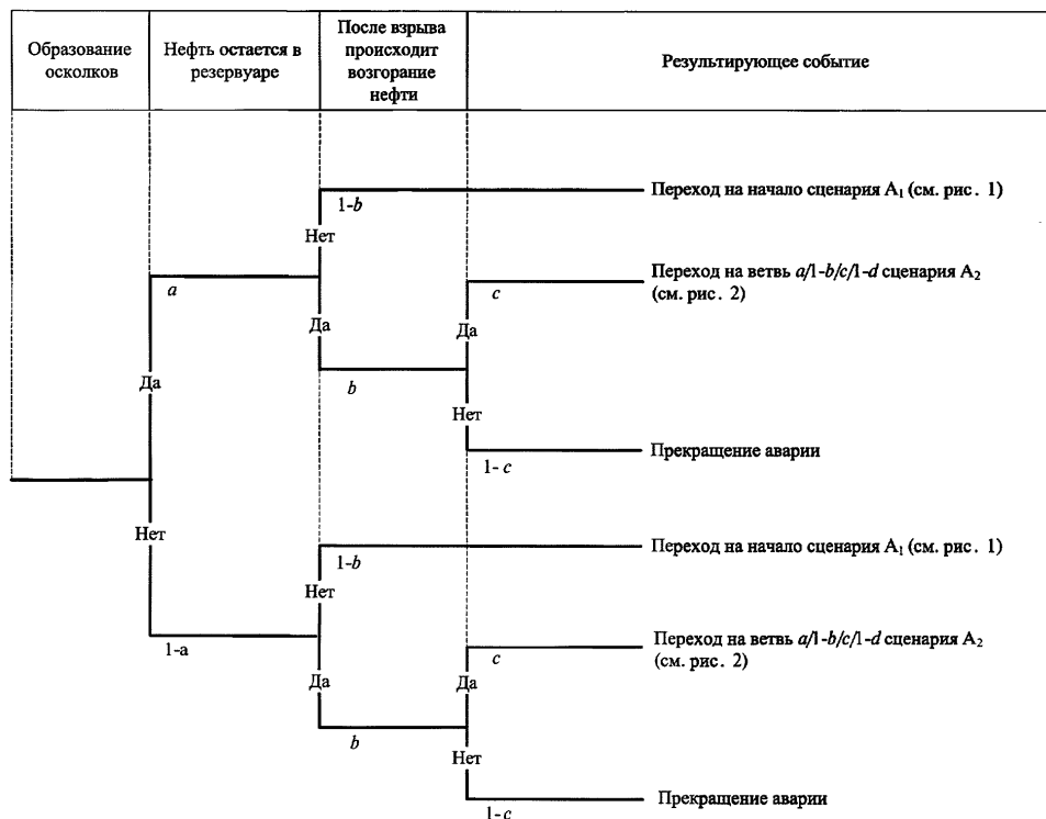
Рис. 3. Дерево событий при взрыве внутри наземного резервуара (сценарий A_3 )
