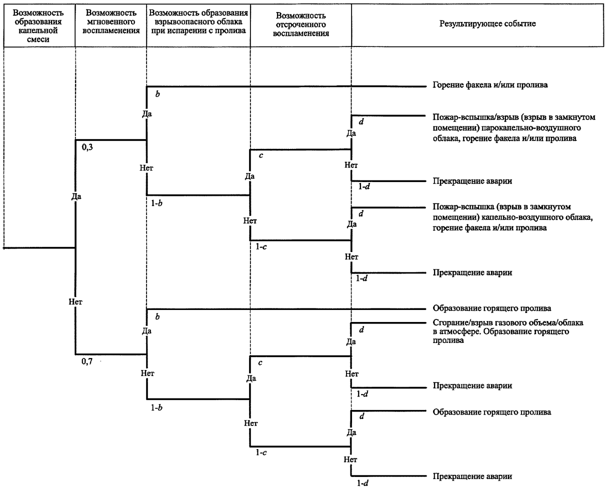
Рис. 9. Дерево событий при аварии в насосных (сценарий A_9 )
