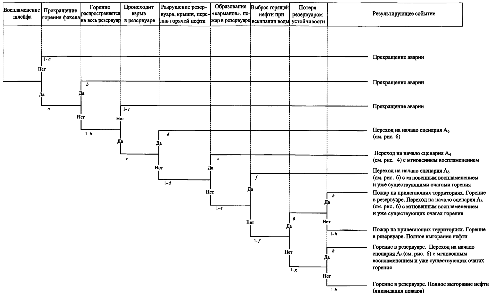
Рис. 5. Дерево событий при выходе газовой фазы из подземного резервуара (типа ЖБР) (сценарий А 2 )
