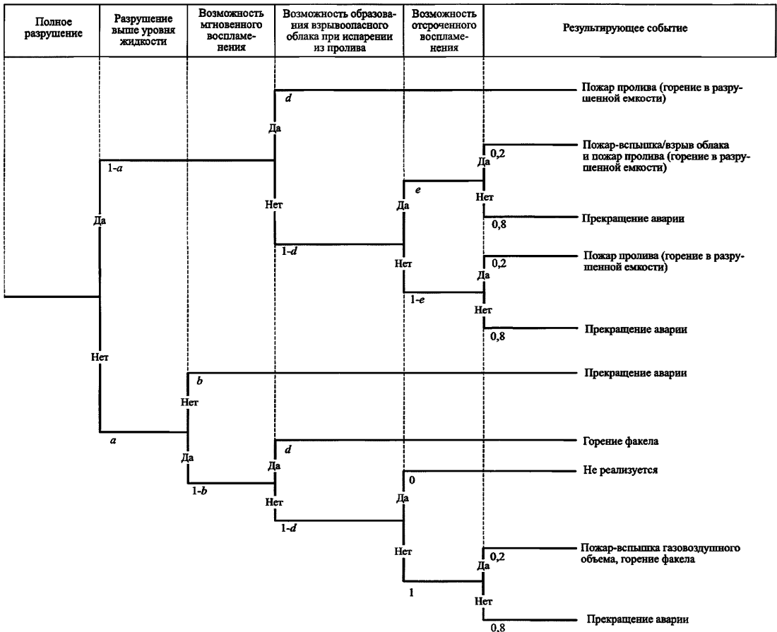
Рис. 8. Дерево событий при разрушении емкости под давлением (сценарий A_3 )
