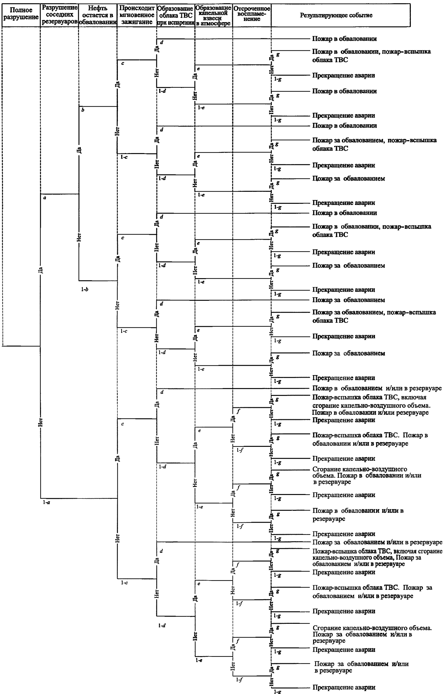
Рис. 1. Дерево событий разрушения/перелива наземного резервуара (сценарий А 1 )
