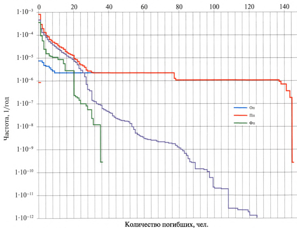
Рис. 10. F/N -диаграмма риска гибели людей от различных аварий на объекте
