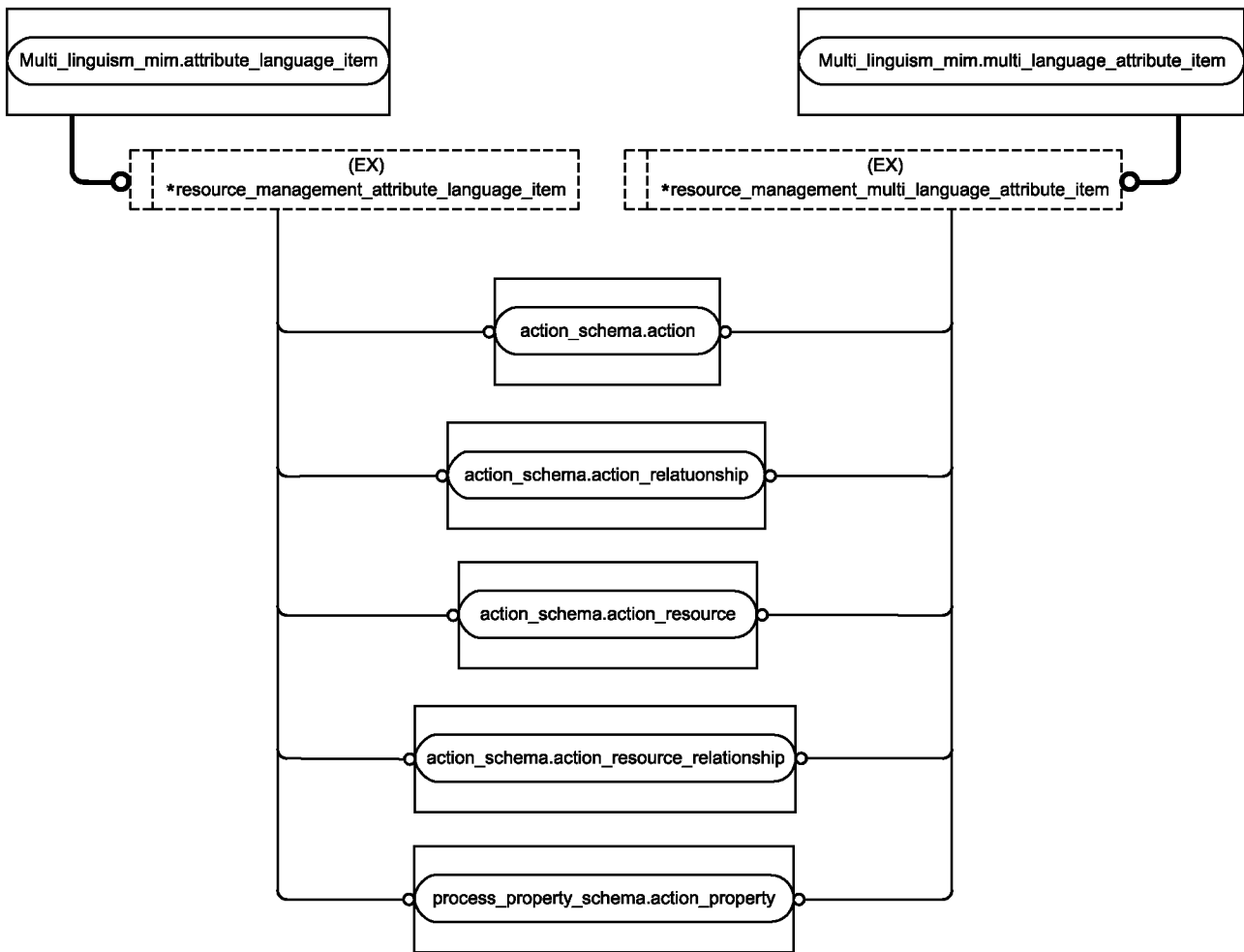
Рисунок D.6 — Представление ИММ на уровне объектов в формате EXPRESS-G (диаграмма 5 из 5)
