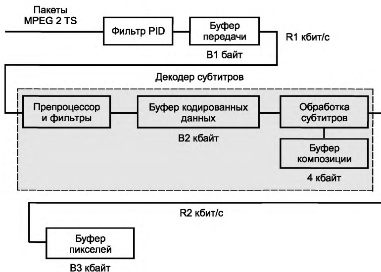
Рисунок 2 — Модель декодера субтитров
