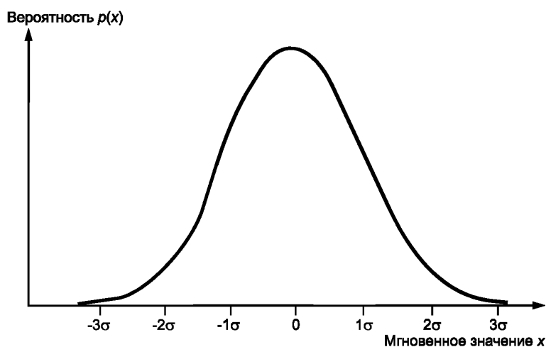
Рисунок 1 — Гауссовская плотность распределения вероятностей
