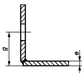
Сварной фланец
