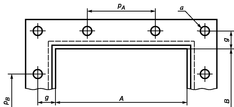
Приваренный внахлест фланец
