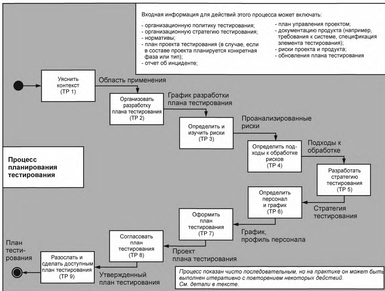
Рисунок 6 — Процесс Планирования Тестирования
