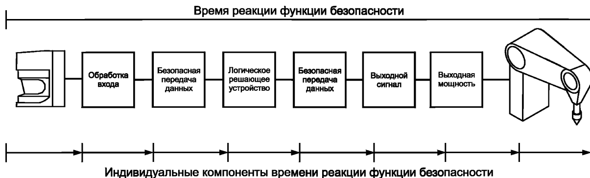
Рисунок 5 — Пример компонентов, составляющих время реакции функции безопасности
