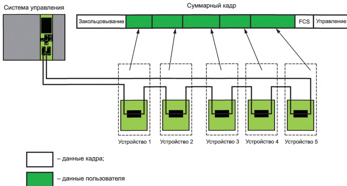
Рисунок 12 — Входные условия для коммуникации FSCP 6/7
