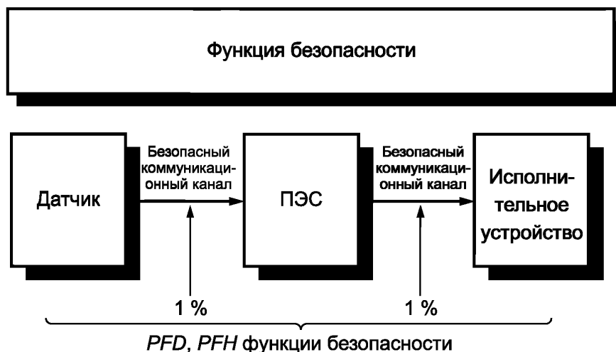
Рисунок 3 — Безопасная коммуникация является частью функции безопасности
