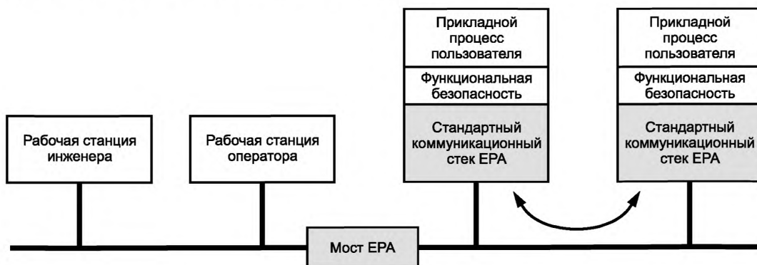
Рисунок 16 — FSCP 14/1 архитектура коммуникации безопасности
