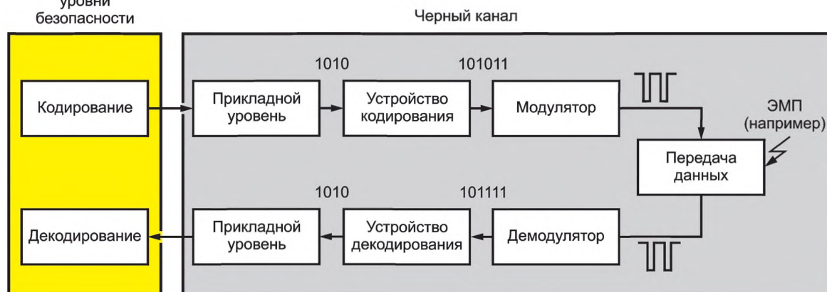
Рисунок В.1 — Коммуникационный канал с искажениями
