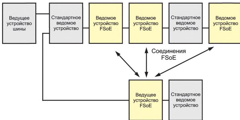
Рисунок 13 — Базовая система FSCP 12/1
