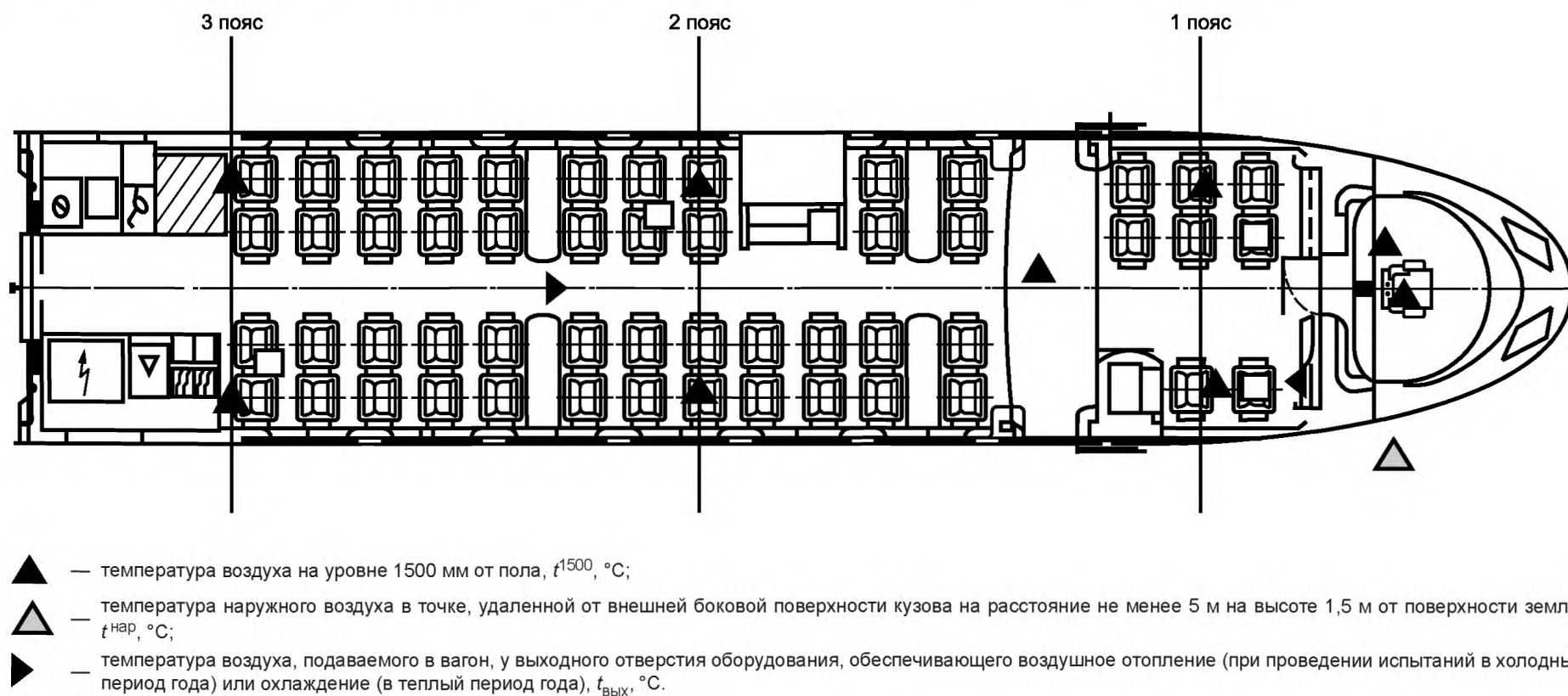
Рисунок И.1 — Размещение точек измерения параметров при проведении испытаний по определению показателей эффективности системы обеспечения микроклимата в кабине и салоне головного вагона
