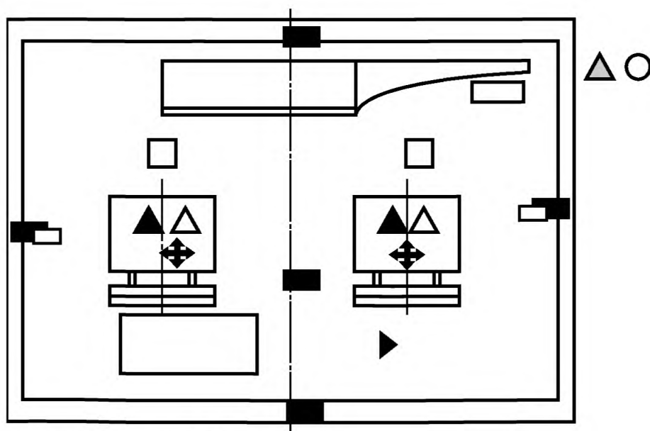
Рисунок Б.12 — Размещение точек измерения параметров микроклимата для холодного периода года в кабине СРС
