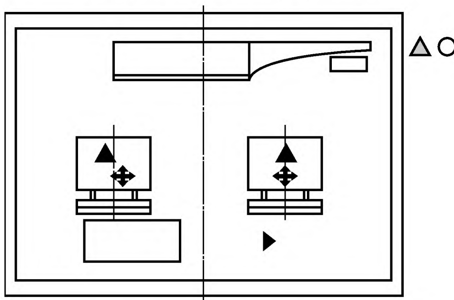
Рисунок Б.5 — Размещение точек измерения параметров микроклимата для теплого периода года в операторской СПС
