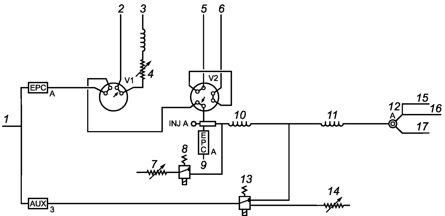
1 — подача гелия; 2 — ввод пробы в жидком состоянии; 3 — выход пробы в жидком состоянии; 4 — игольчатый клапан № 1; 5 — ввод пробы в газообразном состоянии; 6 — выход пробы в газообразном состоянии; 7 — игольчатый клапан № 3; 8 — двухходовой электромагнитный клапан; 9 — выход; 10 — предколонка; 11 — аналитическая колонка для оксигенатов; 12 — FID детектор; 13 — трехходовой электромагнитный клапан; 14 — игольчатый клапан № 2; 15 — вспомогательный газ; 16 — водород; 17 — подача воздуха
