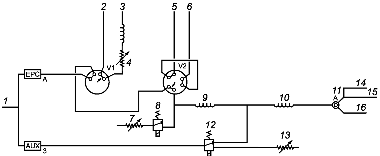
1 — подача гелия; 2 — ввод пробы в жидком состоянии; 3 — выход пробы в жидком состоянии; 4 — игольчатый клапан № 1; 5 — ввод пробы в газообразном состоянии; 6 — выход пробы в газообразном состоянии; 7 — игольчатый клапан № 3; 8 — двухходовой электромагнитный клапан; 9 — предколонка; 10 — аналитическая капиллярная колонка для оксигенатов; 11 — FID детектор; 12 — трехходовой электромагнитный клапан; 13 — игольчатый клапан № 2; 14 — вспомогательный газ; 15 — водород; 16 — подача воздуха
