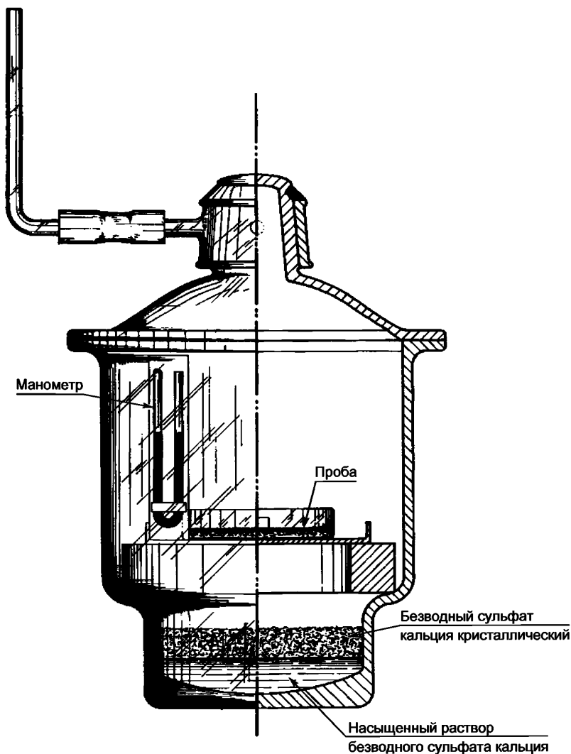
Рисунок 1 — Вакуумный эксикатор
