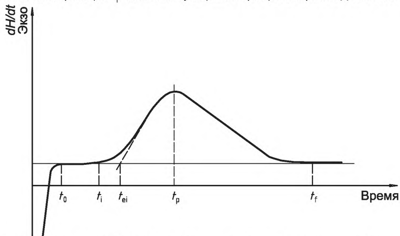
Рисунок 2 — Кривая ДСК с экзотермическим пиком (изотермический метод)
