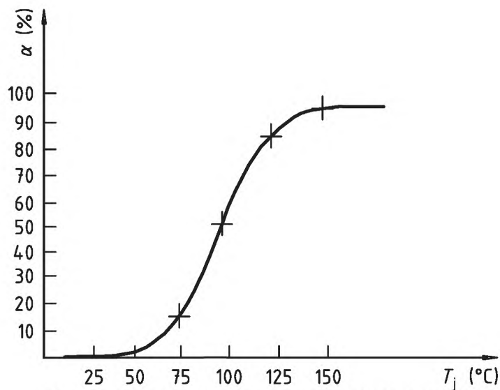
Рисунок 5 — Пример увеличения \alpha с температурой
