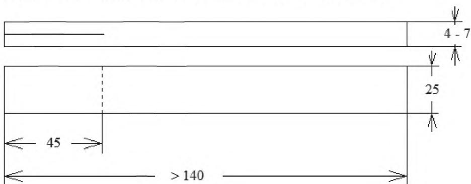
Рисунок 2 – Эскиз образца в форме двухконсольной балки
