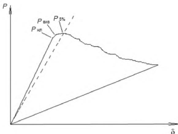
Рисунок 1 – Типовая диаграмма нагрузка – перемещение
