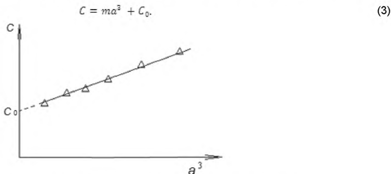
Рисунок 4 – Зависимость податливости образца от длины трещины
