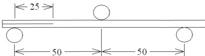
Рисунок 5 – Начальное положение образца на испытательной оснастке
