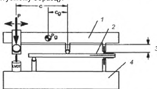
1 – рычаг; 2 – образец испытаний; 3 – погрузочная высота; 4 – основание Рисунок 1 – Оснастка для испытаний по смешанной моде нагружения I + II
