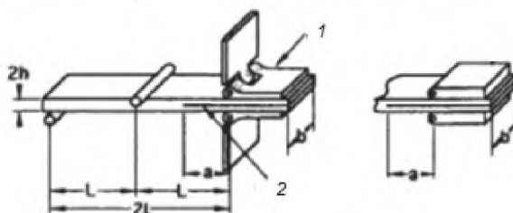
1 – шарнир; 2 – расслаивание
