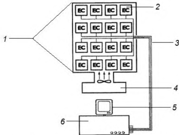
1 — плоскость испытания 1220 × 1830 мм; 2 — стекла с ЭХП; 3 — электрические выводы и кабели термпар; 4 — термшкаф; 5 — компьютер; 6 — многоканальная цифровая автоматизированная система управления и сбора данных
