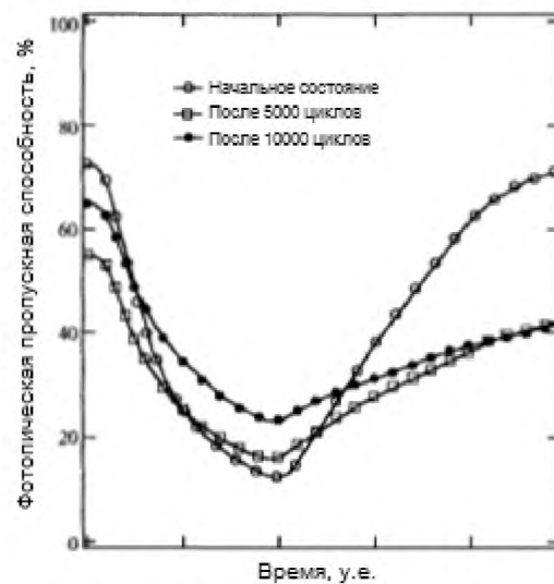
Рисунок 5 — Фотооптическая пропускная способность как функция времени, измеренного на различных этапах циклических испытаний типового окна с ЭХП
