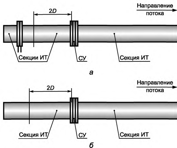
а — прямолинейный участок ИТ изготовлен из нескольких секций; б — прямолинейный участок ИТ изготовлен из одной секции
