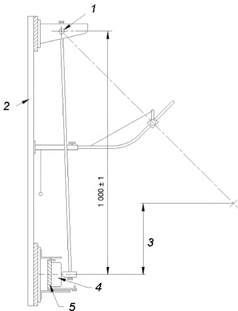
Рисунок 1 — Маятниковый стенд для испытаний на ударные воздействия
