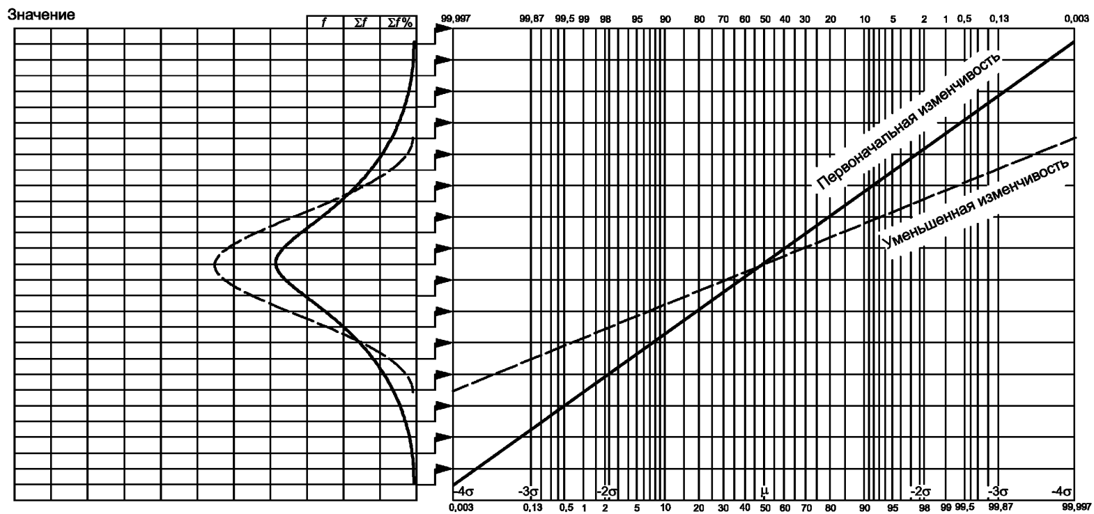
Рисунок 4 — Слишком большая изменчивость. Машина после улучшений
