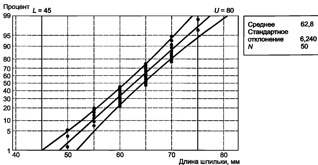
График функции распределения вероятностей для длины шпилек, мм Нормальное распределение Доверительный интервал уровня 95 %
