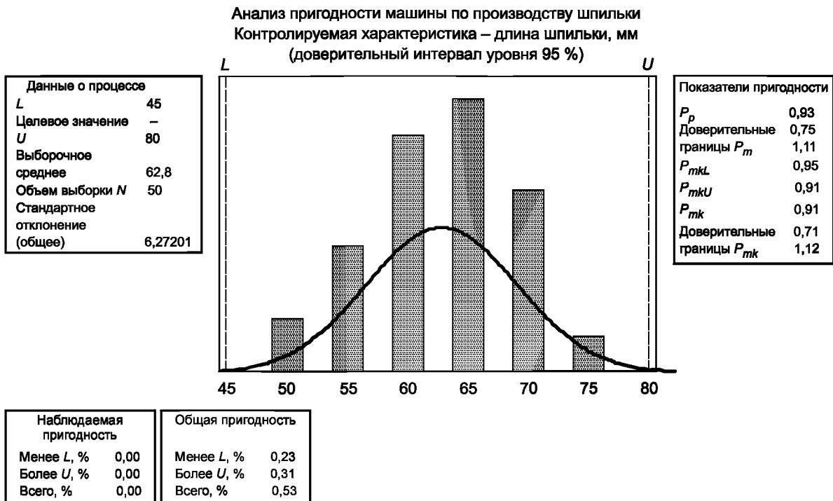
Рисунок В.2 — Пример результатов исследований пригодности машины
