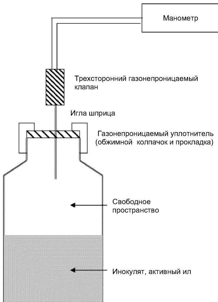
Рисунок 1 — Прибор для определения образования биологического газа по давлению газа
