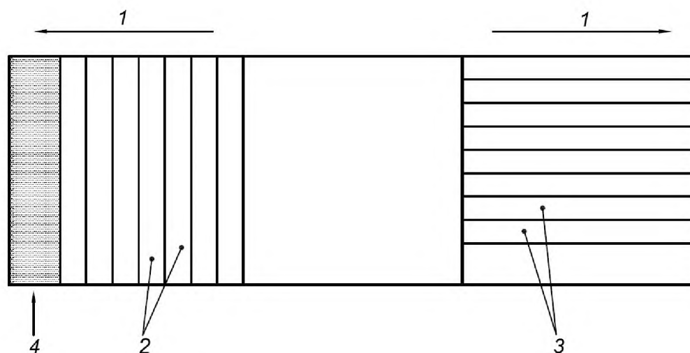
1 — направление текучести; 2 — образцы, перпендикулярные к направлению текучести; 3 — образцы, параллельные направлению текучести; 4 — брак
