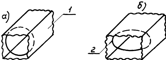
Рис. 6. Схема установки внутренних вставок жесткости: а - кольцевой; б - овальной
