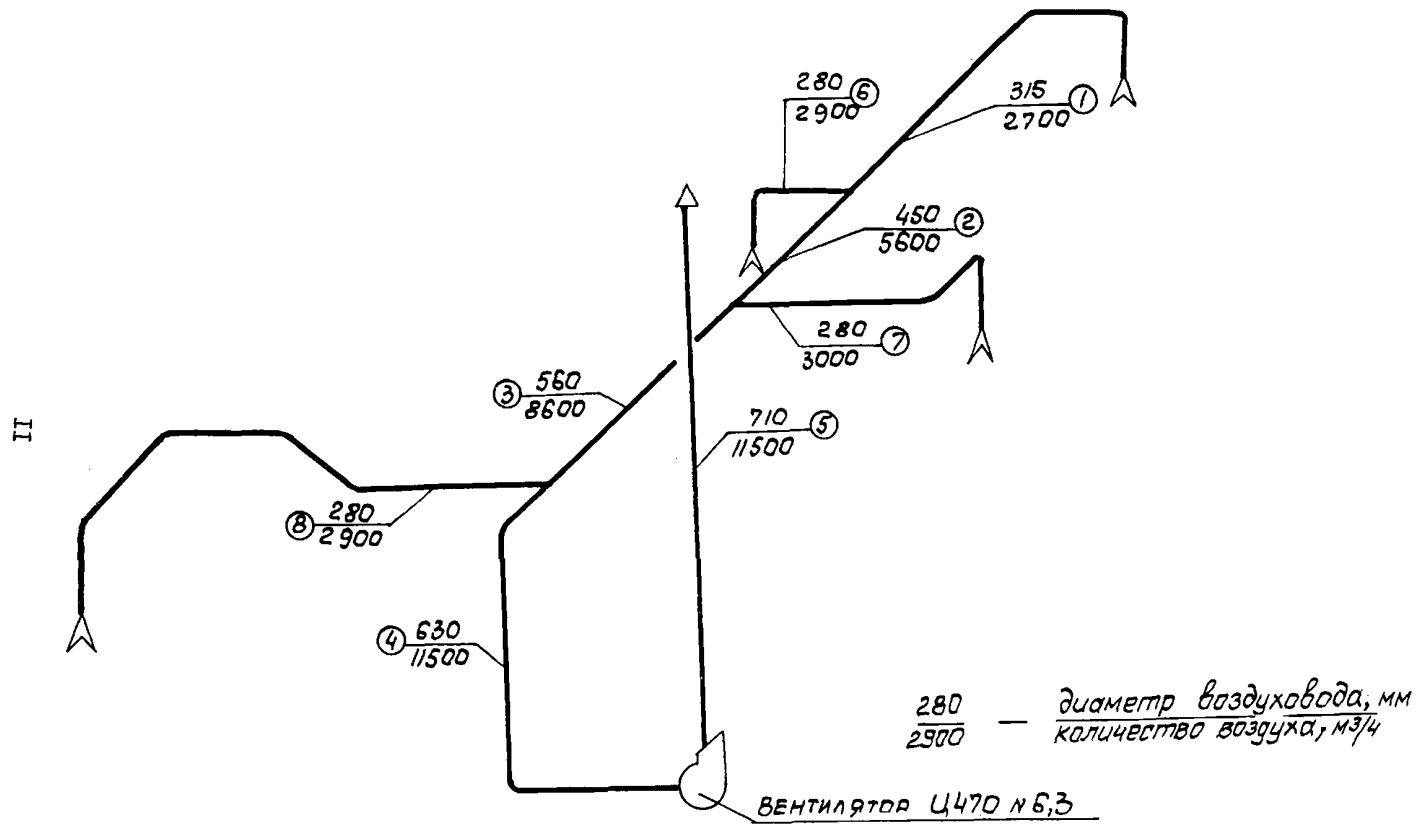
Рис.1. Расчетная схема сети воздуховодов вытяжной системы вентиляции общего назначения
