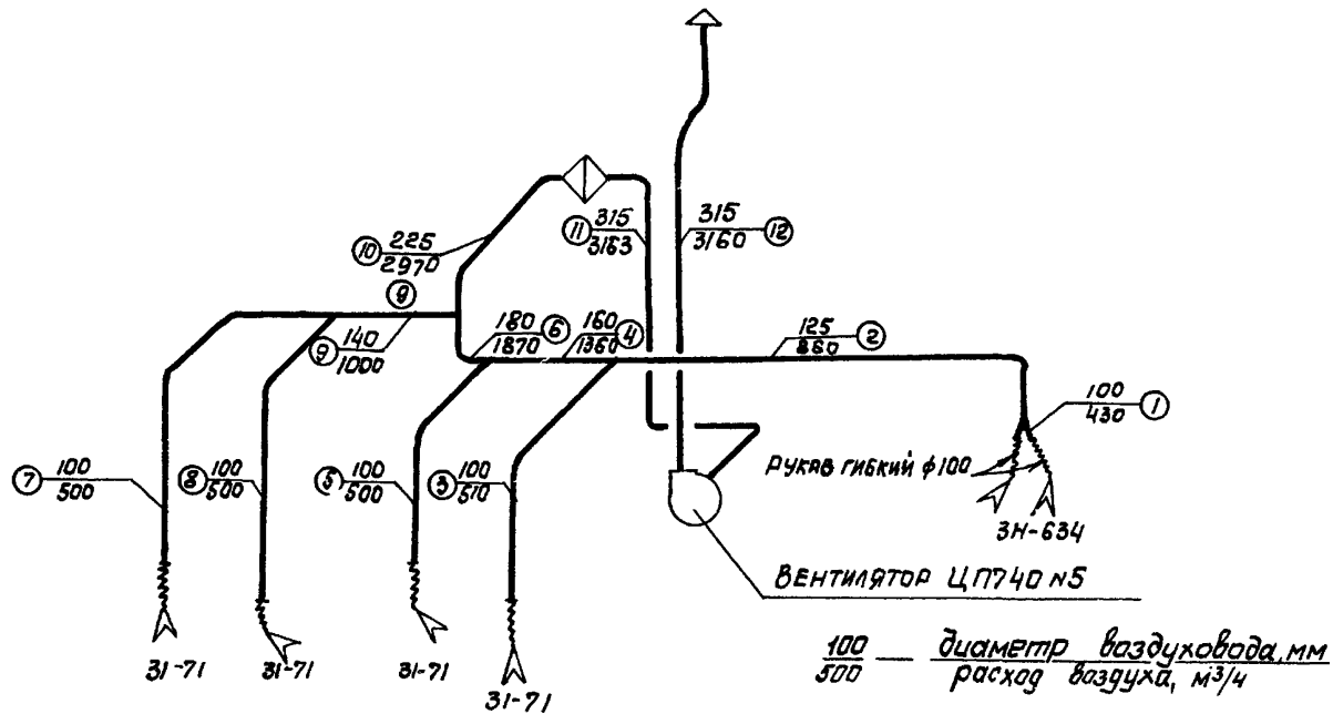
Рис.3. Расчетная схема сети воздуховодов системы аспирации
