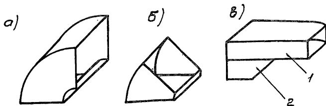
Рис.2 Отводы прямоугольного сечения:
