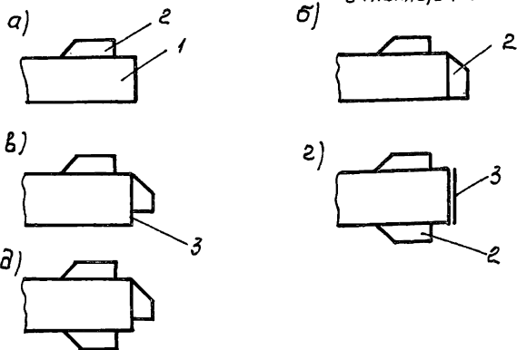
Рис.3. Схема образования узлов ответвления прямоугольного сечения:
