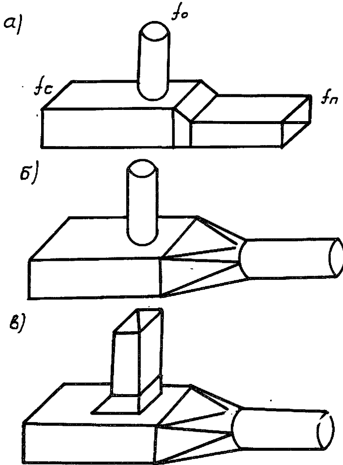
Рис. 4.-Узлы ответвления вентиляционных комбинированных систем со стволом прямоугольного сечения
