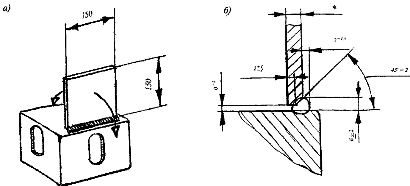
Рис. 3.1 Специальная тавровая проба, испытываемая на излом:
