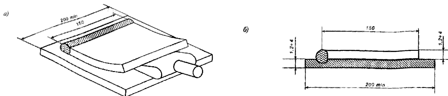
Рис. 3.4 Наклесточная проба, испытываемая на разъединение пластин:
