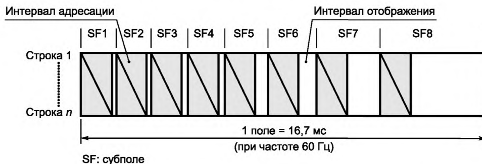
Рисунок А.8 — Метод разделения интервала адресации и интервала отображения
