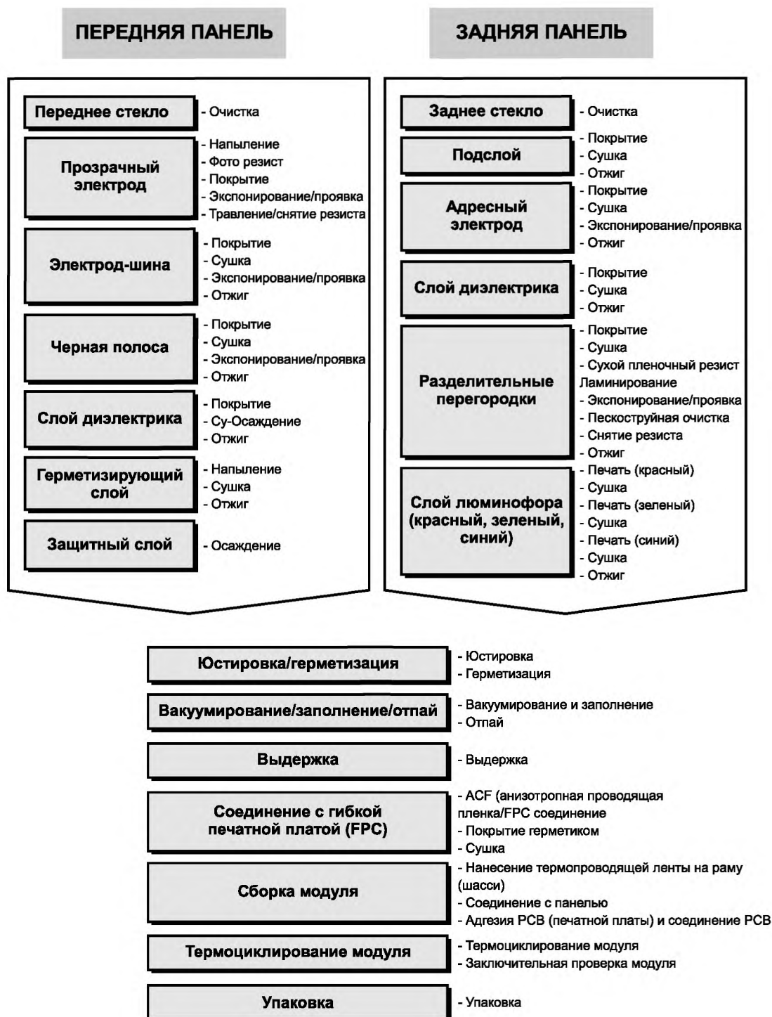
Рисунок D.1 — Алгоритм производства (изготовления) PDP
