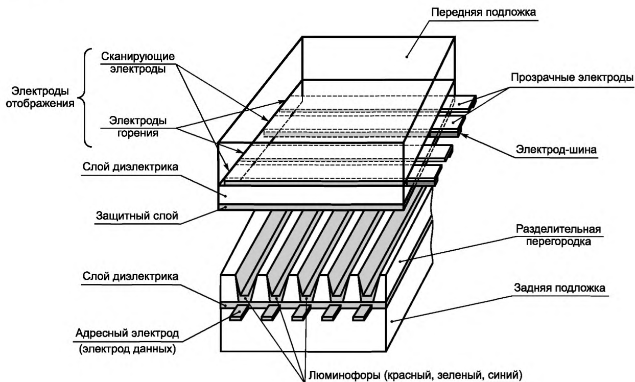
Рисунок А.7 — Структура цветной АС PDP трехэлектродного типа и поверхностным разрядом
