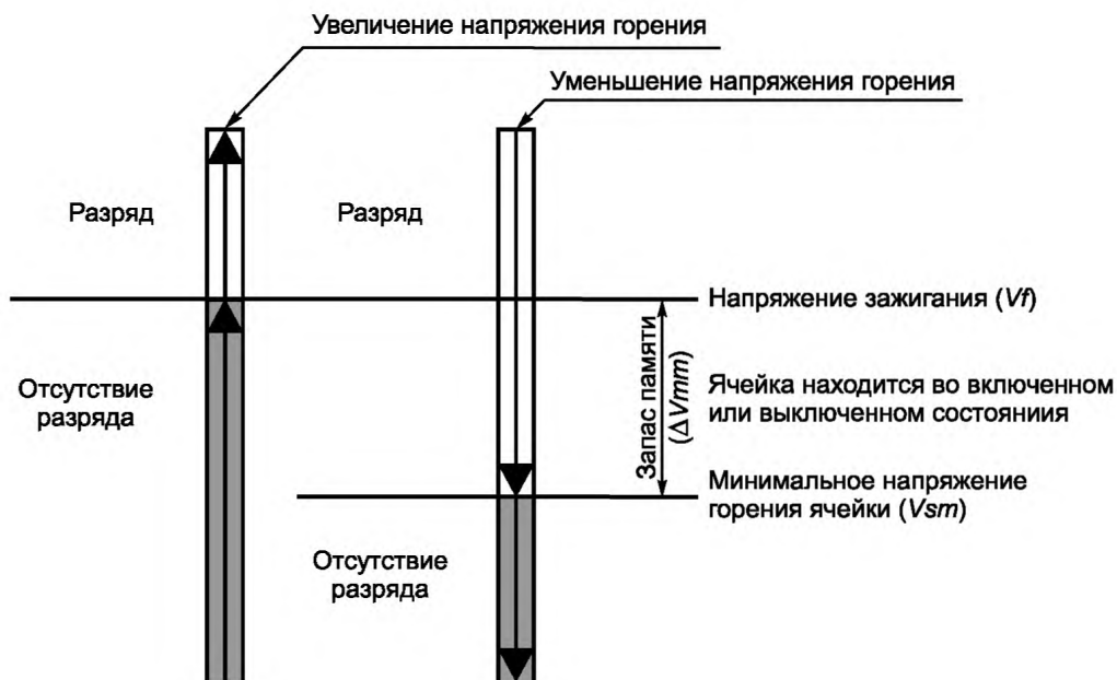
Рисунок А.2 — Разрядные характеристики ячейки (статические характеристики единичной ячейки)
