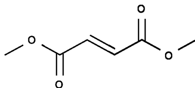
Рисунок В.4 — Молекулярная структура диметилфумарата
