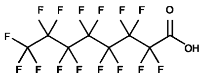
Рисунок В.11 — Молекулярная структура ПФОК
