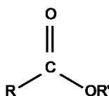
Рисунок А.2 — Эфирная связь
