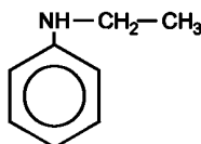
Рисунок В.7 — Молекулярная структура Н-этилфениламина
