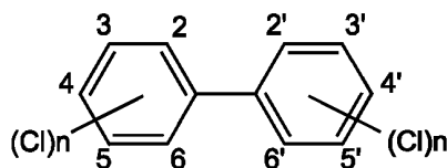
Рисунок В.13 — Молекулярная структура ПХБФ
