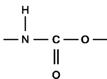
Рисунок А.1 — Уретановые группы
