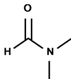
Рисунок В.3 — Молекулярная структура ДМФА
