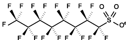
Рисунок В.10 — Молекулярная структура ПФОС
