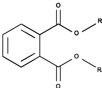
Рисунок В.12 — Молекулярная структура фталатов
