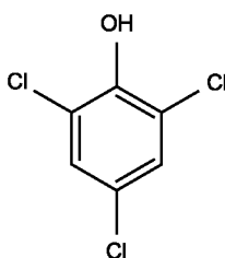
Рисунок В.14 — Молекулярная структура и номер по CAS полихлорфенолов
