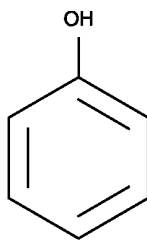
Рисунок В.18 — Структура фенола
