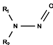
Рисунок В.8 — Молекулярная структура нитрозаминов
