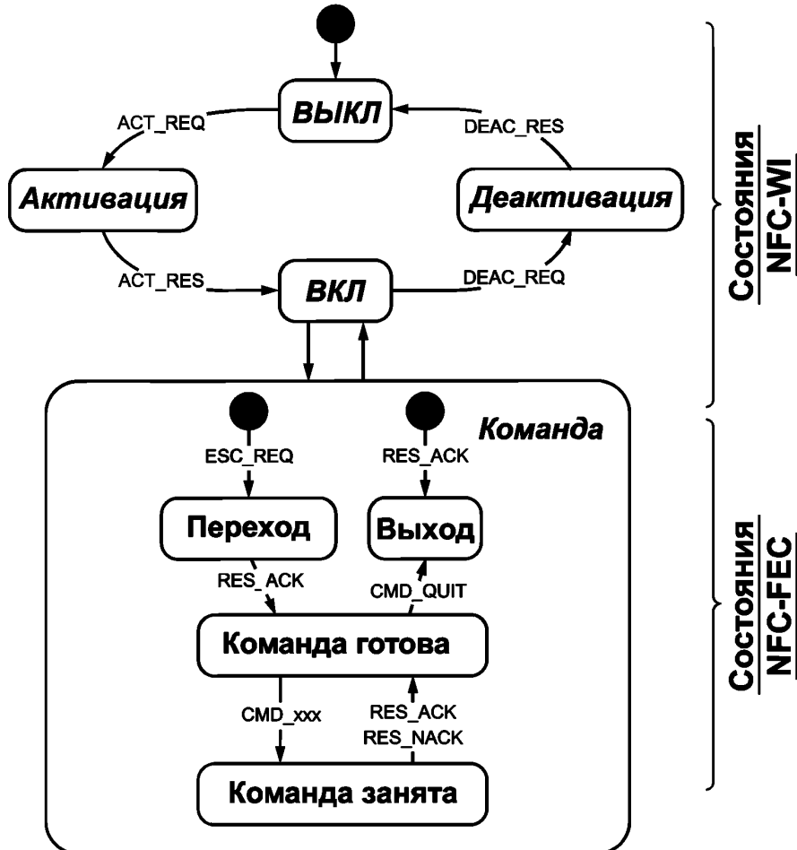
Рисунок 1 — Состояния NFC-WI и подсостояния NFC-FEC
