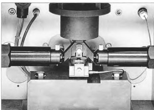
Рисунок 2 – Испытательная камера
