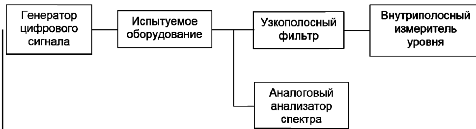
Рисунок 7 — Схема соединения оборудования
