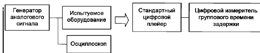
Рисунок 20 — Схема соединения оборудования
