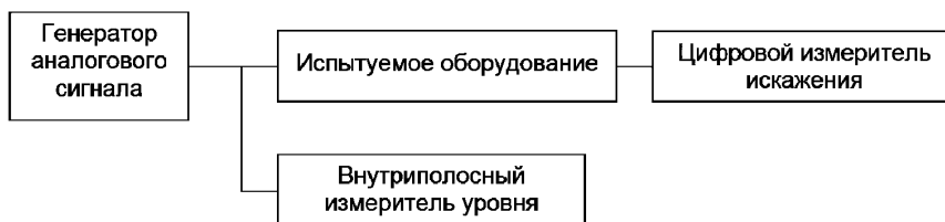
Рисунок 33 — Схема соединения оборудования
