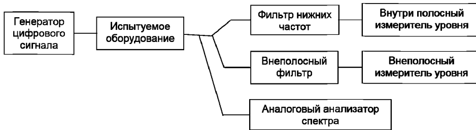
Рисунок 6 — Схема соединения оборудования
