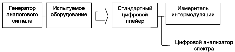
Рисунок 36 — Схема соединения оборудования
