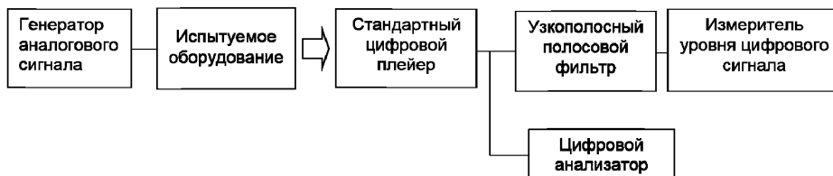
Рисунок 28 — Схема соединения оборудования
