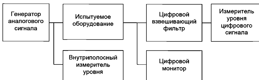
Рисунок 21 — Схема соединения оборудования
