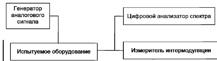
Рисунок 35 — Схема соединения оборудования
