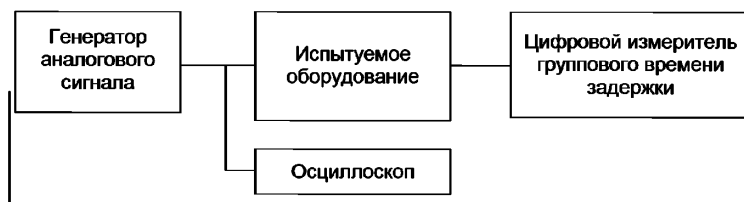
Рисунок 19 — Схема соединения оборудования
