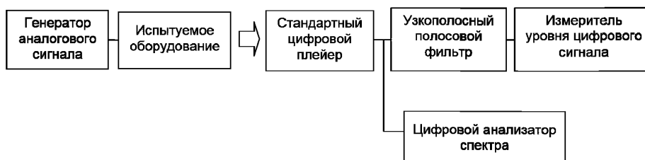
Рисунок 30 — Схема соединения оборудования
