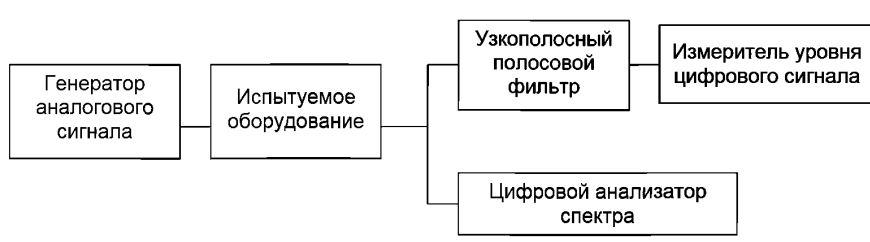
Рисунок 29 — Схема соединения оборудования
