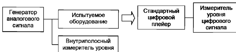
Рисунок 26 — Схема соединения оборудования
