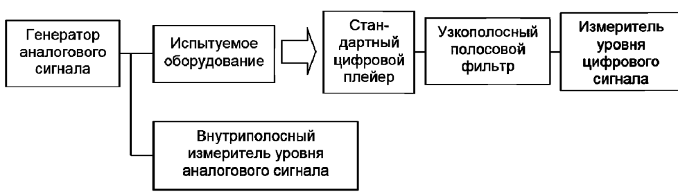
Рисунок 32 — Схема соединения оборудования
