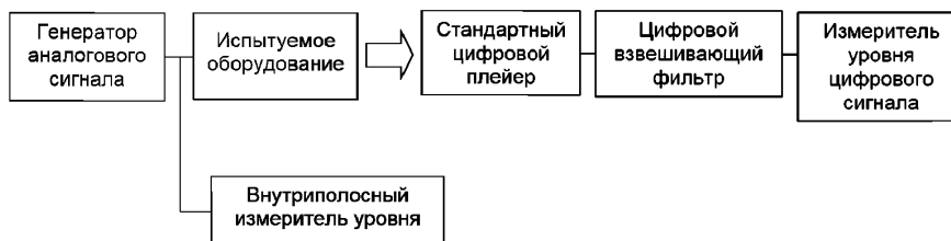
Рисунок 22 — Схема соединения оборудования
