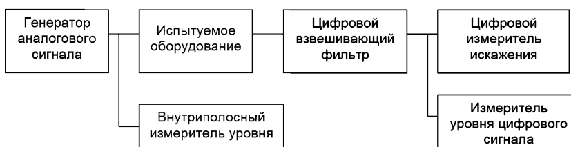
Рисунок 23 — Схема соединения оборудования
