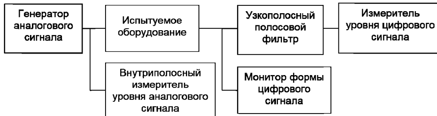
Рисунок 31 — Схема соединения оборудования
