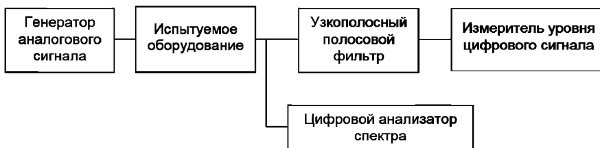
Рисунок 27 — Схема соединения оборудования
