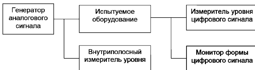
Рисунок 17 — Схема соединения оборудования
