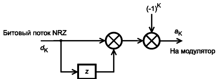
Рисунок 2 — Блок-схема предварительного кодера GMSK
