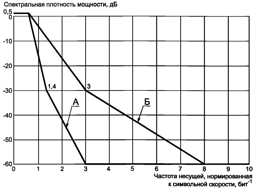
Кривая А — спектральная маска для информативности передачи данных более 2 Мбит/с. Кривая Б — спектральная маска для информативности передачи данных менее 2 Мбит/с.
