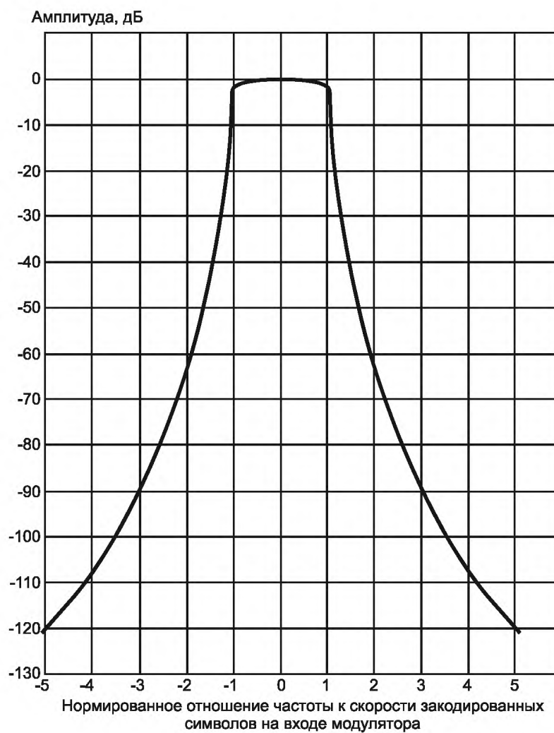
Рисунок 9 — АЧХ фильтра Баттерворта 6-го порядка
