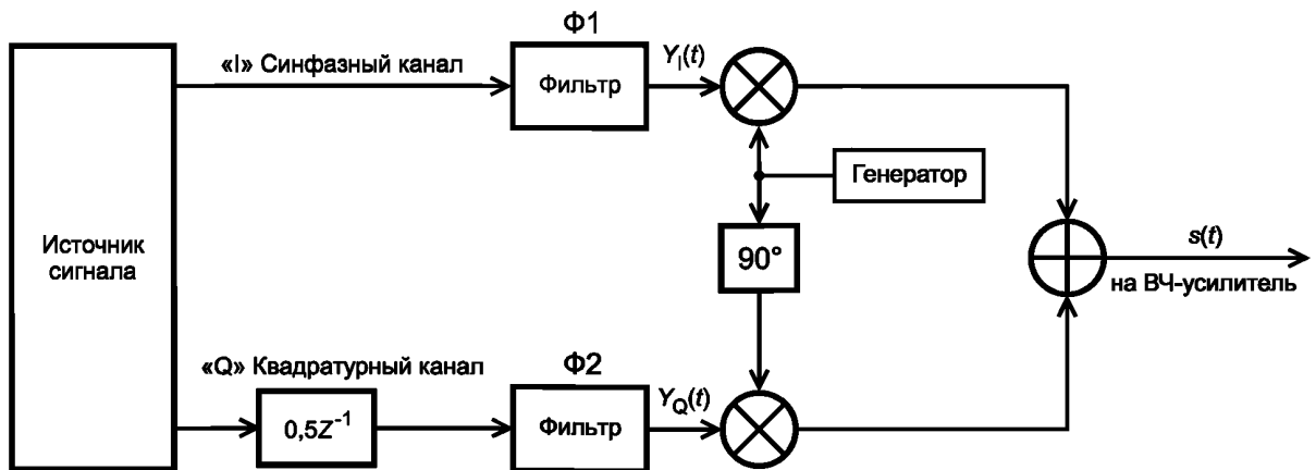
Рисунок 7 — Блок-схема квадратурно-синфазного модулятора с фильтрацией основной полосы частот
