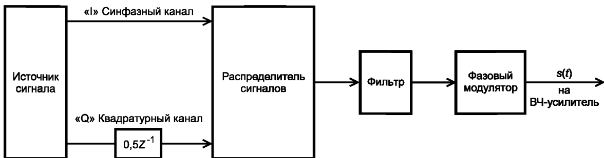
Рисунок 5 — Блок-схема линейного фазового модулятора OQPSK
