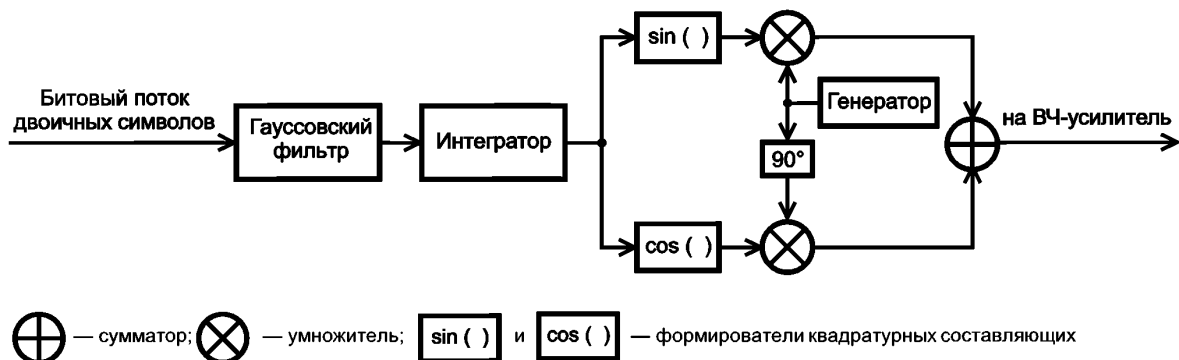
Рисунок 4 — Блок-схема квадратурного модулятора GMSK с фазовым сдвигом
