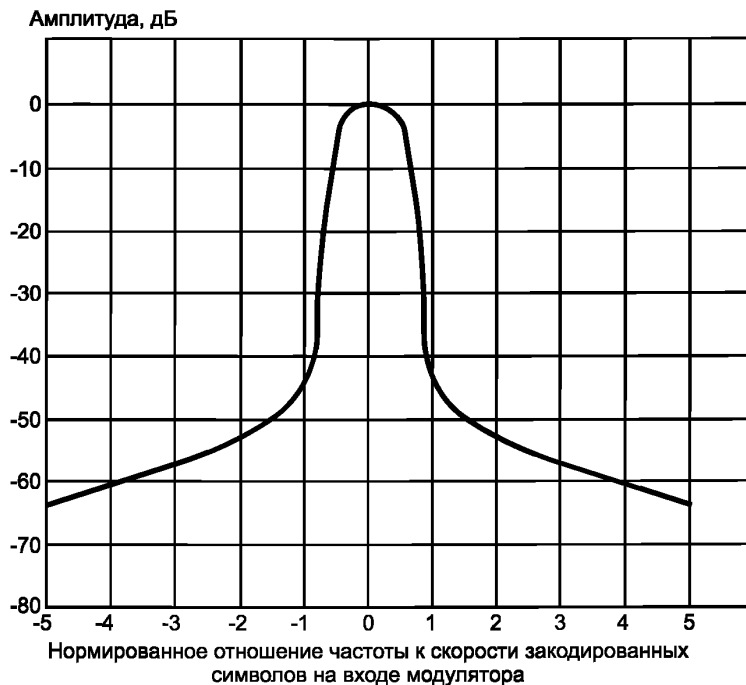
Рисунок 11 — Вид АЧХ фильтра SRRC при \alpha = 0,5
