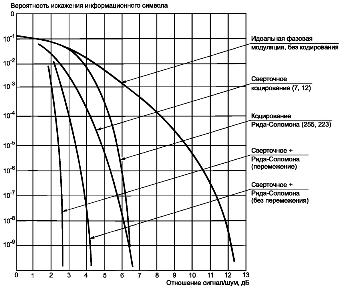
Рисунок А.1 — Графическая зависимость вероятности искажения информационного символа от величины отношения сигнал/шум E_b/N_0 при различных методах помехоустойчивого кодирования
