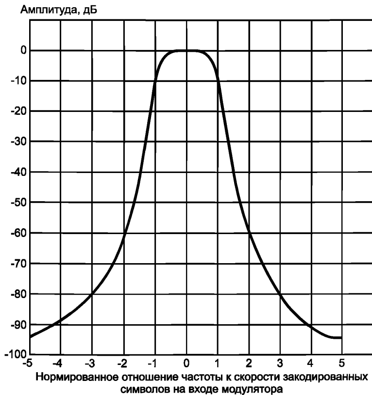
Рисунок 14 — АЧХ фильтра Бесселя 6-го порядка
